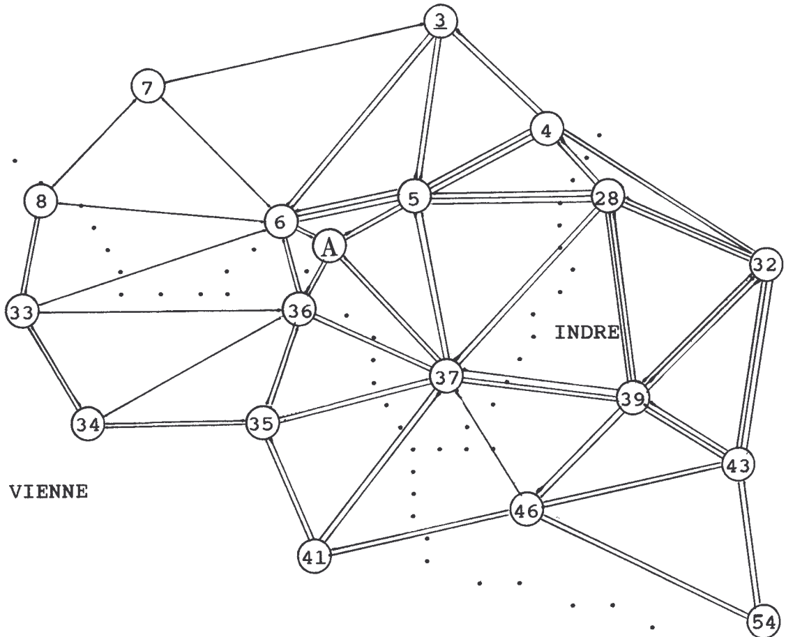
Carte des interpoints en fonction des co-identités
