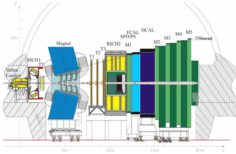
FIGURE 2: Disposition du détecteur LHCb dans le plan y - z [4]
