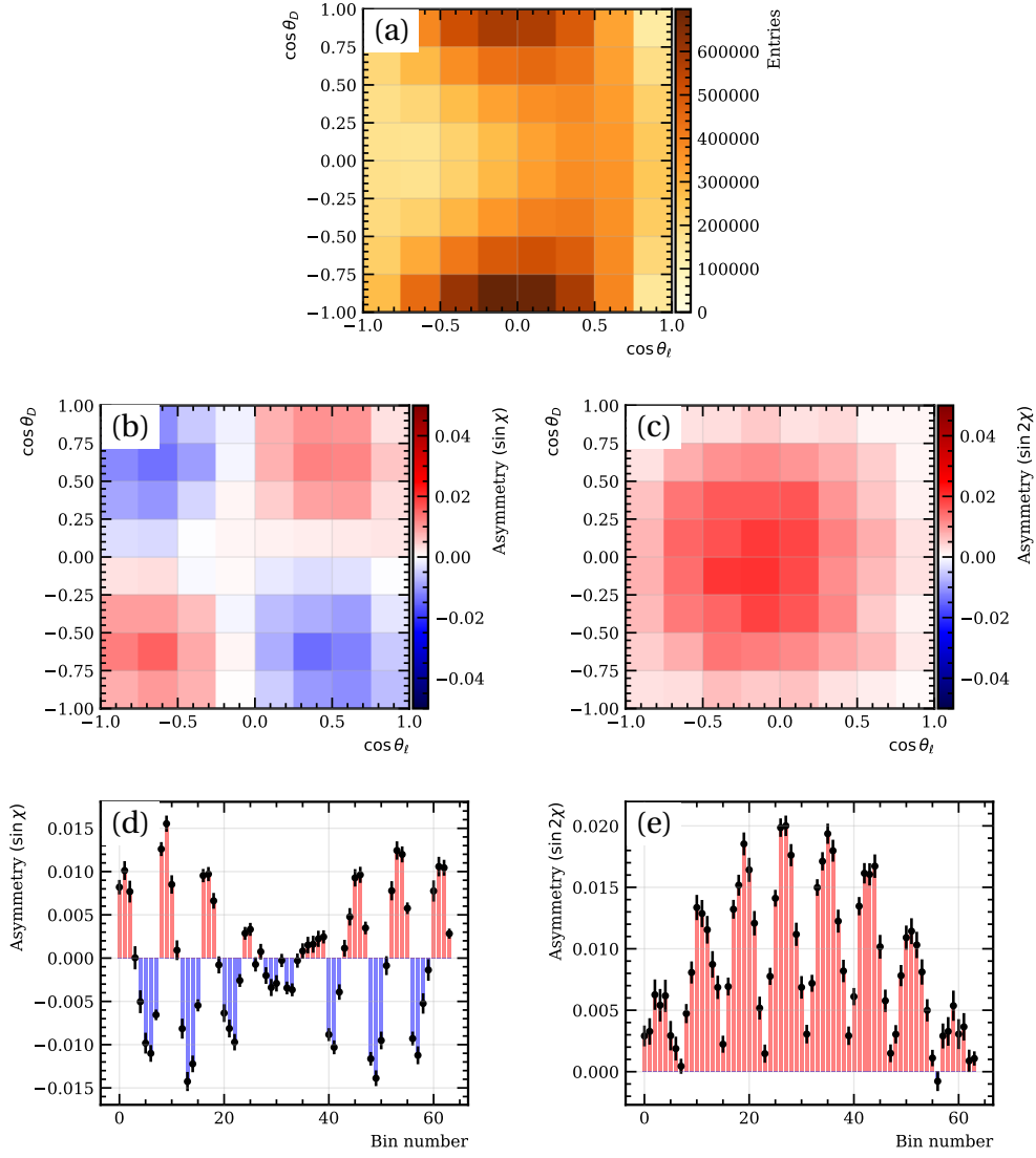
FIGURE 3: Densité des événements (a), asymétries CP 2D (b,c) et asymétries CP 1D (d,e) des termes \sin\chi et \sin 2\chi dans les variables (\cos\theta_D, \cos\theta_\ell) intégrés sur q^2 dans le cas NP de \text{Im}(g_R) = 0, 1i .
