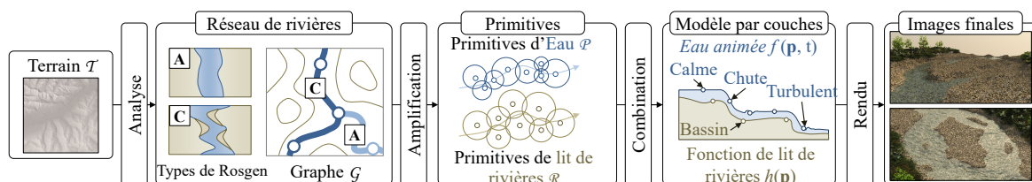
FIGURE 2 : Présentation de la méthode : l'entrée est un champ de hauteur 2D à partir duquel les caractéristiques d'écoulement sont automatiquement dérivées. Un réseau fluvial et une géométrie du lit sont construits en utilisant la catégorisation de Rosgen (Figure 3). Ensuite, les paramètres d'écoulement dérivés pour chaque cellule de la rivière sont transmis à un processus d'amplification procédurale. Le résultat est un modèle de rivière sous la forme d'un arbre de construction qui encode une fonction temporelle d'élévation de l'eau w(\mathbf{p}, t) .
