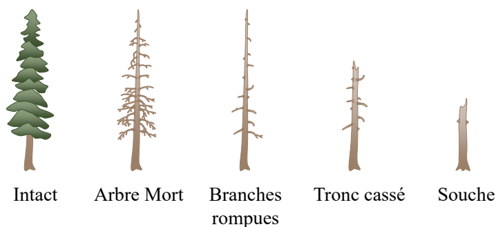
FIGURE 25 : Les cinq stades de décomposition suivant la mort de l’arbre, utilisés pour classer les arbres morts sur pied (chicots).
