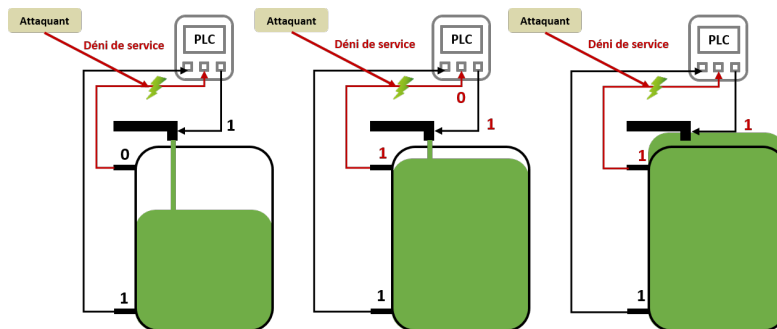
FIGURE 3.18 – Manipulation du programme PLC par blocage
