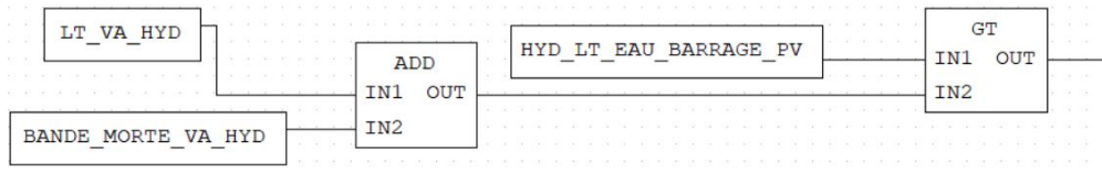
FIGURE 3.14 – Exemple d'un réseau FBD
