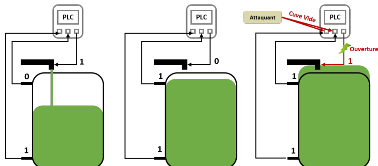
FIGURE 3.19 – Manipulation du programme PLC par forçage
