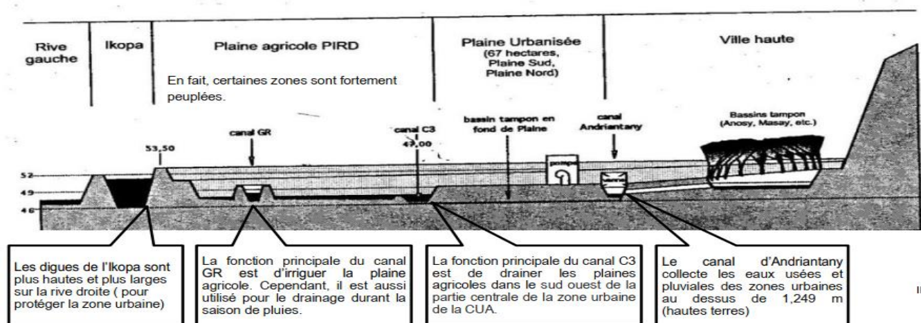
Figure 3 : Système de protection et de drainage (PIRD : Périmètre Irrigé de la Rive Droite de l'Ikopa) (Source : PUDi, 2019)
