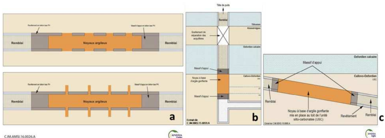
Figure 4 – Les zones de scellements utilisant des bétons dans Cigéo : a- deux options pour les alvéoles MAVL et les galeries ; b- puits ; c- descendrière (IRSN, 2017 d'après ANDRA).
