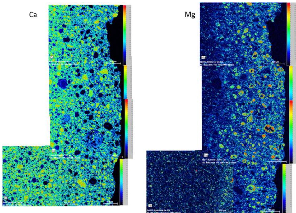
Figure 22 – Série de cartographies EDS du calcium et du magnésium le long de la surface de la pâte de ciment bas-pH (T3 L ) après 2 mois d'immersion dans une solution représentative de l'eau naturelle de l'oxfordien calcaire.
