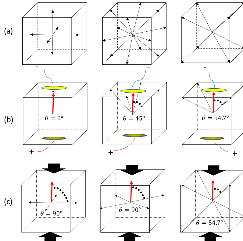
FIGURE 4: Les différentes orientations possibles de la polarisation pour les phases tétraogonaux, orthorhombiques et rhomboédriques (de gauche à droite). (a) Configurations possibles sans champ électrique et contrainte appliqués ; (b) Configurations possibles lorsqu'un champ électrique est appliqué ; (c) Configurations possibles lorsqu'une contrainte uniaxiale est appliquée. Les flèches rouges représentent le champ électrique et les flèches noires représente la contrainte.
