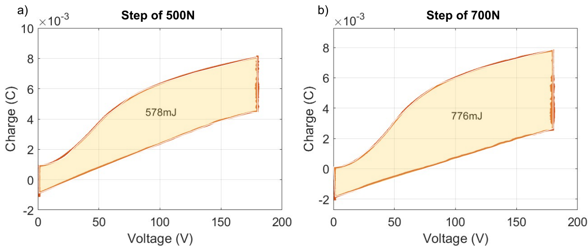
FIGURE 11: Cycles d'Ericsson avec des vrais pas; (a) 500N; (b) 700N.
