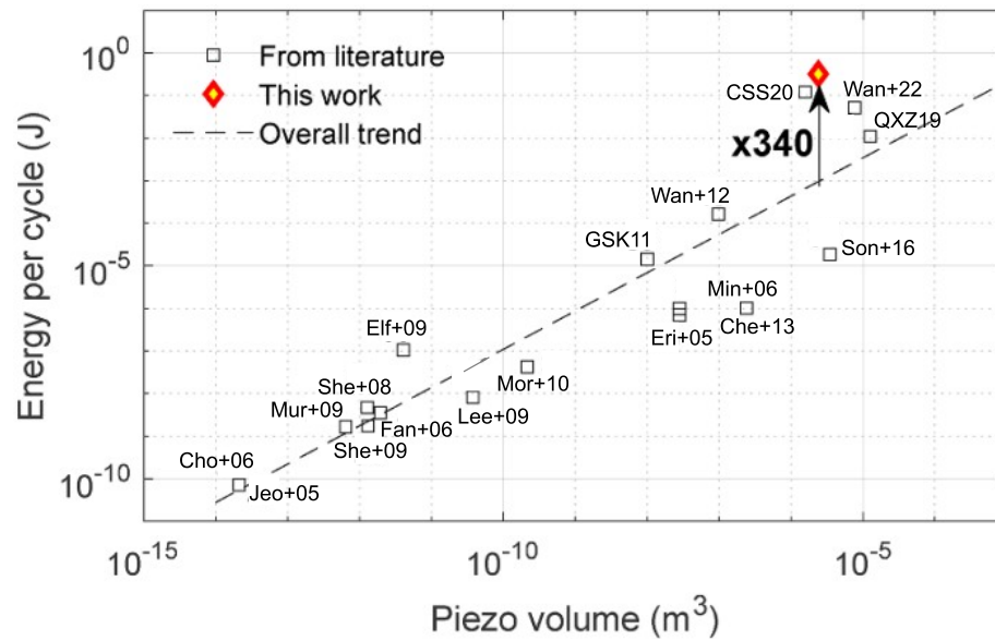
FIGURE 13: Tendance générale de l'énergie de sortie des dispositifs de récupération d'énergie piézoélectrique en fonction du volume des éléments piézoélectriques [Seb+23].
