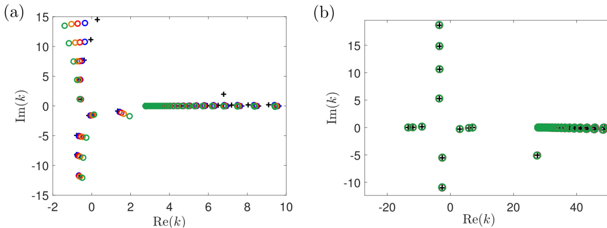
FIGURE 8.7 – Nombres d’onde des modes de conduit pour un écoulement avec un nombre de Mach de 0.3 et pour une fréquence normalisée de (a) 0.93 et (b) de 9.3, calculés à partir (+) des équations d’Euler linéarisées et (o) avec une suppression graduelle du terme de gradient (la suppression complète correspond au vert). Extrait de Ref. [58].
