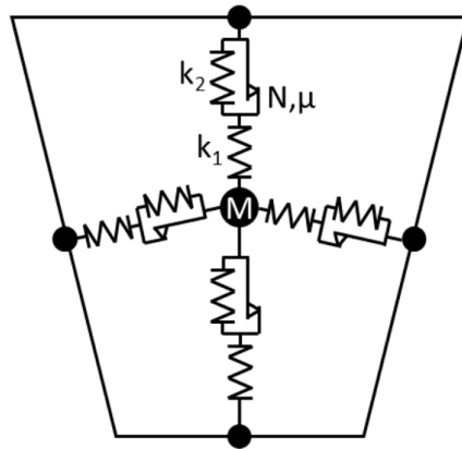
FIGURE 3.37 – Systèmes de Masing entre la masse centrale et les nœud maîtres des parois d'un caisson
