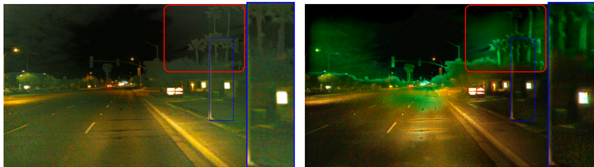
(f) EnlightenGAN
