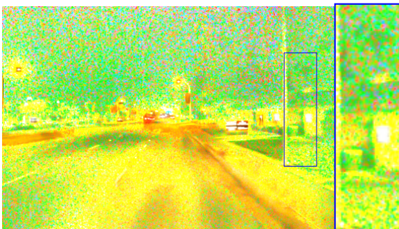
(j) LIME
