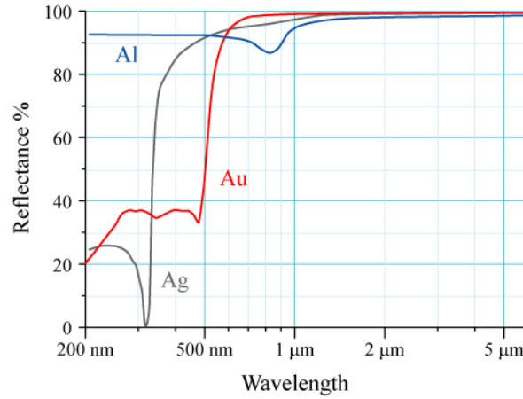
Figure 2: Exemples de spectres de réflectance de métaux. Source : Wikipedia
