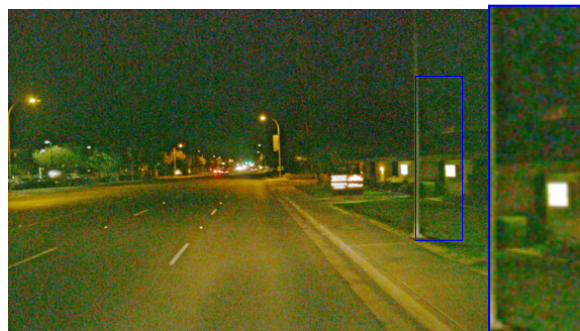
(k) Zero-DCE
