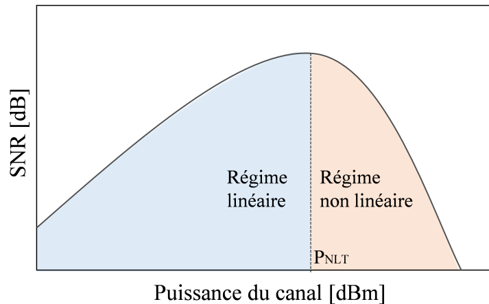
Fig. B.3: Le SNR en fonction de la puissance du canal pour un système de transmission arbitraire.
