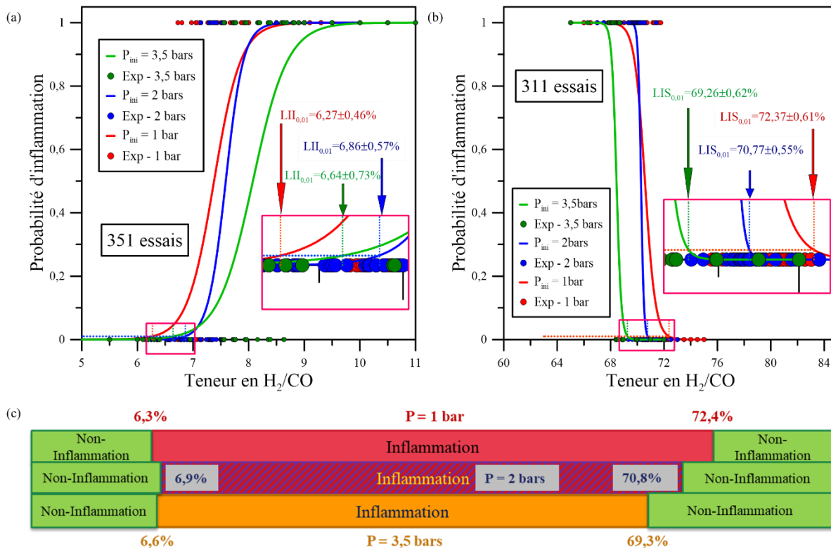
Figure 54 – Comparaison des domaines d'inflammabilité du mélange H 2 /CO/Air déterminés pour les trois pressions initiales étudiées (1 ; 2 ; 3,5 bars) pour T ini = 294,9 ± 0,61 K, et E inflammation = 265 ± 38 mJ. (a) : Limites d'inflammabilité inférieures. (b) : Limites d'inflammabilité supérieures. (c) : Domaines d'inflammabilité complets.
