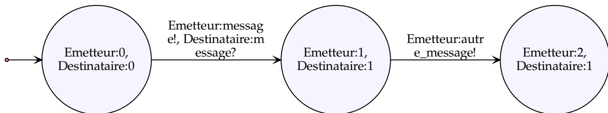
FIGURE 3.7 – Produit synchronisé des automates des composants Emetteur et Destinataire
