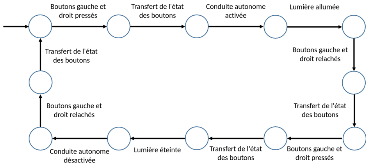
FIGURE 3.23 – Représentation sous forme d’automate du fonctionnement raffiné de l’ISW
