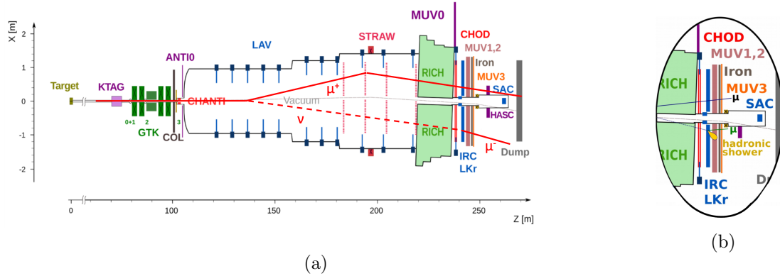
Figure 3.: Schéma de la désintégration K\mu\nu^* superposé à la vue topologique schématique de l'expérience NA62 (4.1a) et un zoom sur les sous-détecteurs qui contribuent à détecter l'interaction du neutrino (4.1b).
