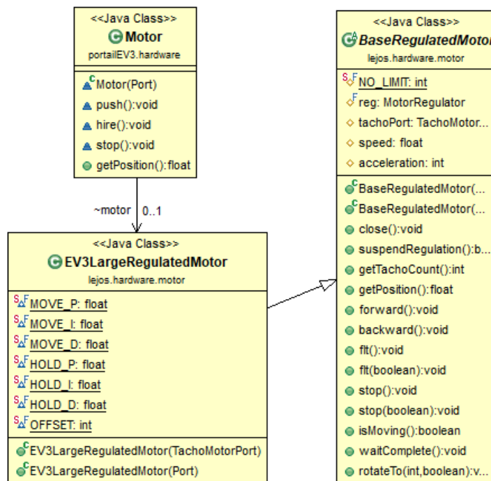
FIGURE 4.14 – Liaison de la classe Motor par adaptation
