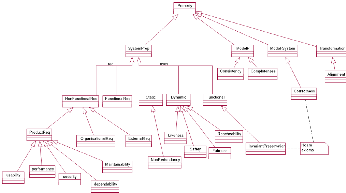
FIGURE 1.8 – Petite taxonomie des propriétés
