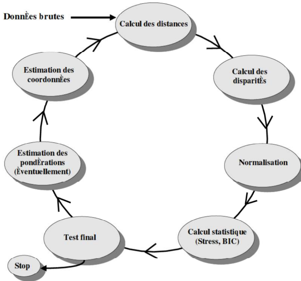
FIG. 4.1 – Algorithme principal de calcul de l'analyse multidimensionnelle.
