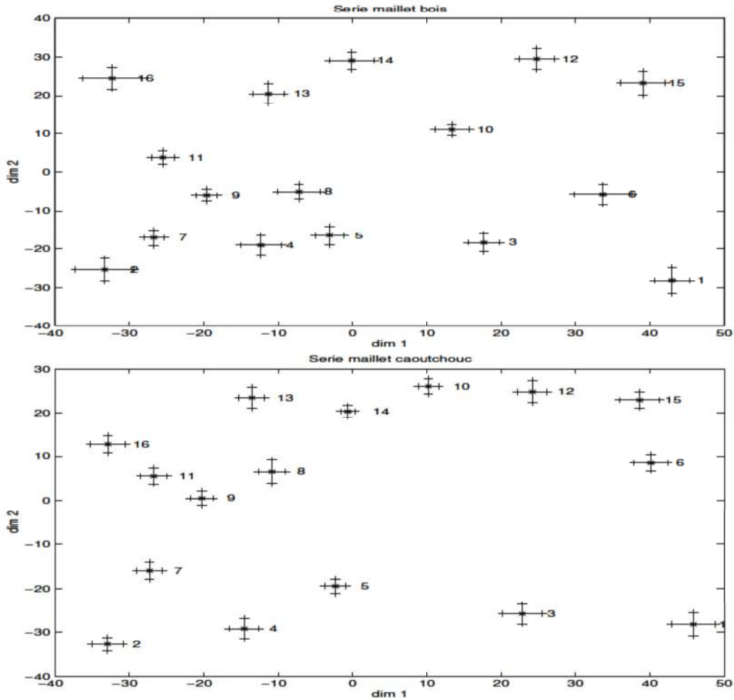
FIG. 9.7 – Espaces perceptifs correspondant aux deux premières dimensions rendues par l'analyse MDS pour les deux séries de sons (maillet bois en haut, maillet caoutchouc en bas). Les écarts-types ont été calculés par la procédure bootstrap sur 250 tirages (la répartition des points est dans l'annexe A, figures A.1 et A.2).
