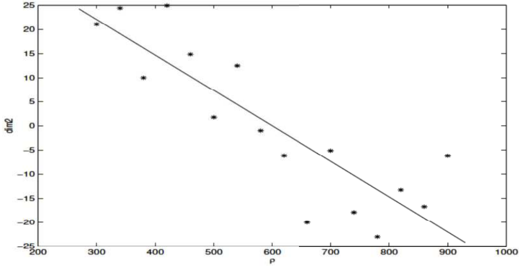
FIG. 7.10 – Représentation de la corrélation entre la dimension perceptive dim2 et la densité du matériau \rho
