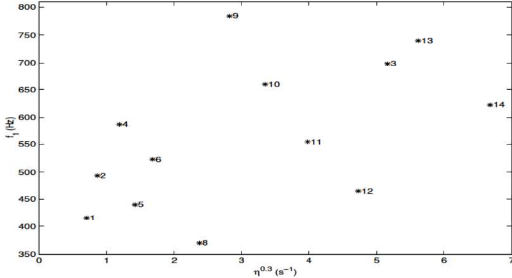
FIG. 8.2 – Espace physique des stimuli. Les paramètres variés sont la fondamentale et le paramètre d'amortissement \eta .
