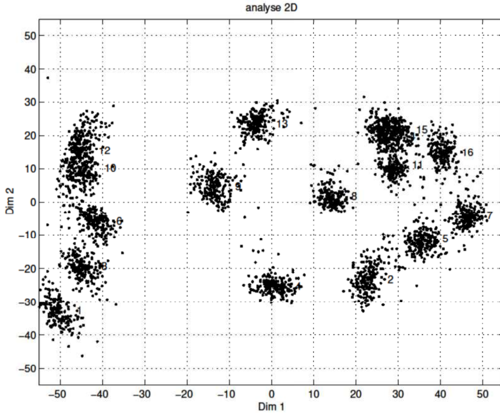
FIG. 4.2 – Nuages de points pour 250 tirages.
