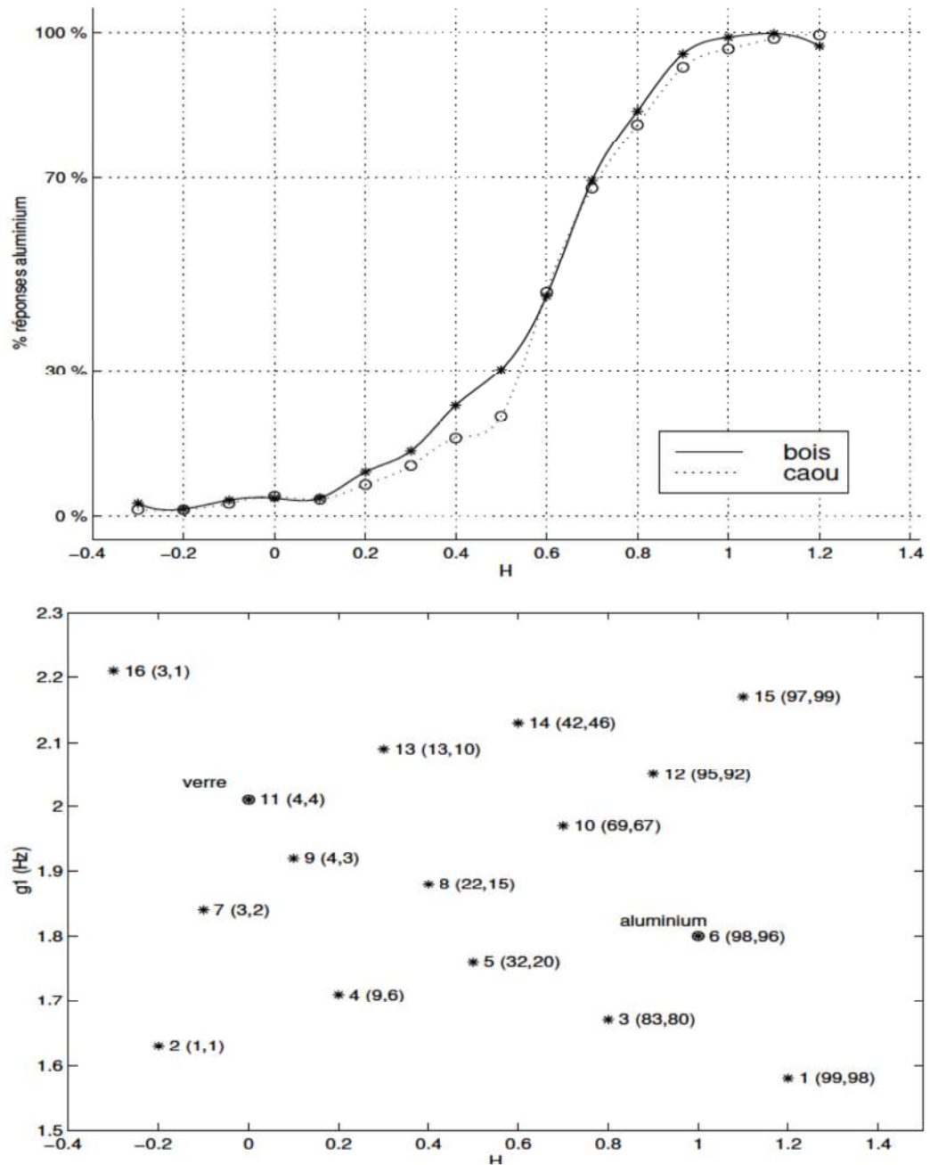
FIG. 9.11 – En bas, espace physique des stimuli indiquant le pourcentage de réponses aluminium (maillet bois, maillet caoutchouc) pour chaque stimulus. En haut pourcentage de réponses en fonction du paramètre d'interpolation H. Seule la dimension 1 correspondant à l'amortissement est utilisée dans les jugements.
