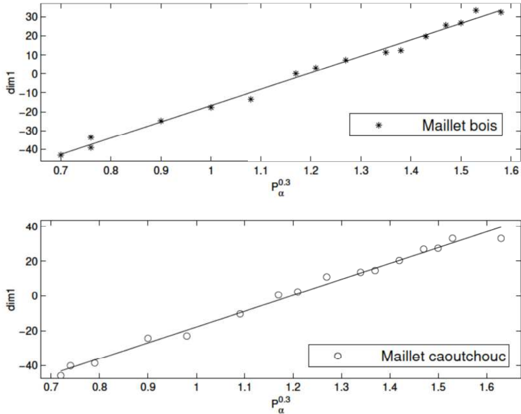
FIG. 9.8 – Corrélation entre P_\alpha^{0.3} , paramètre analytique représentant la pente de la courbe \alpha_i(f) et la dimension perceptive dim1 .
