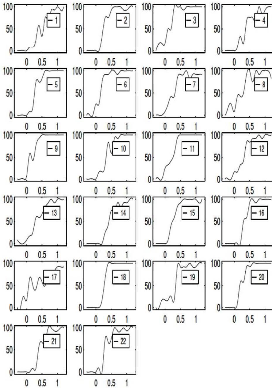
FIG. C.2 – Résultats individuels des sujets numérotés dans la légende pour la série caoutchouc, chaque courbe représente le pourcentage de réponses "aluminium" en fonction du paramètre d'amortissement H .
