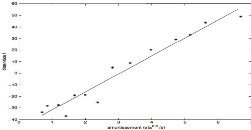
FIG. 8.5 – Représentation de la corrélation entre la dimension perceptive dim1 et le paramètre d'amortissement \eta .
