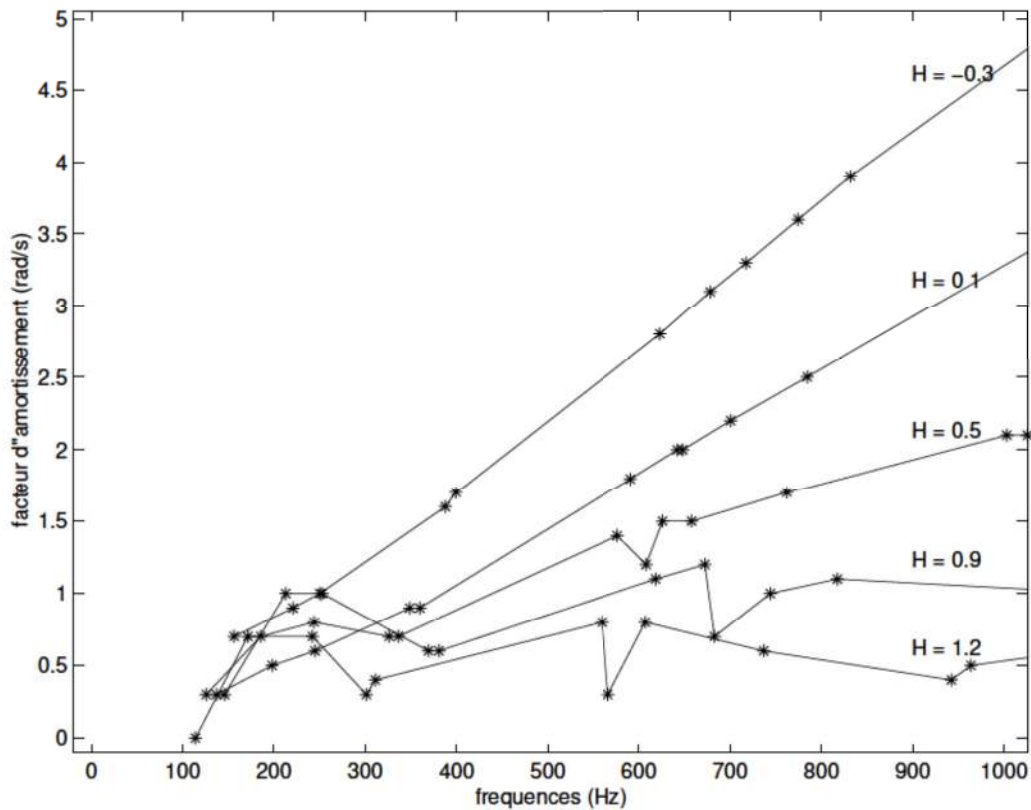
FIG. 9.4 – Représentation des facteurs d'amortissement calculés pour chaque mode et pour 5 stimuli du moins amorti (le bas de la figure) jusqu'au plus amorti (le haut de la figure). Les courbes sont annotées du facteur d'interpolation H introduit dans le modèle hybride d'amortissement.
