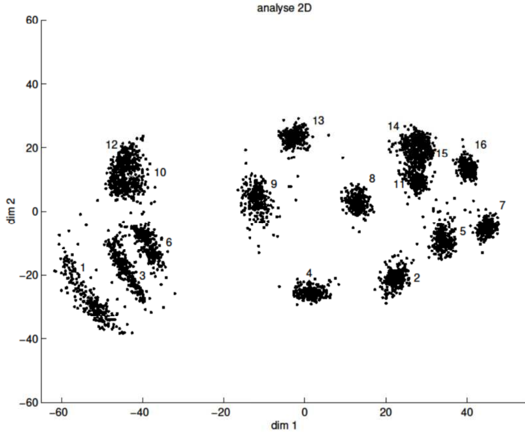
FIG. 7.5 – Représentation des nuages de sons dans l'espace perceptif, le calcul est fait par la méthode bootstrap sur 250 tirages
