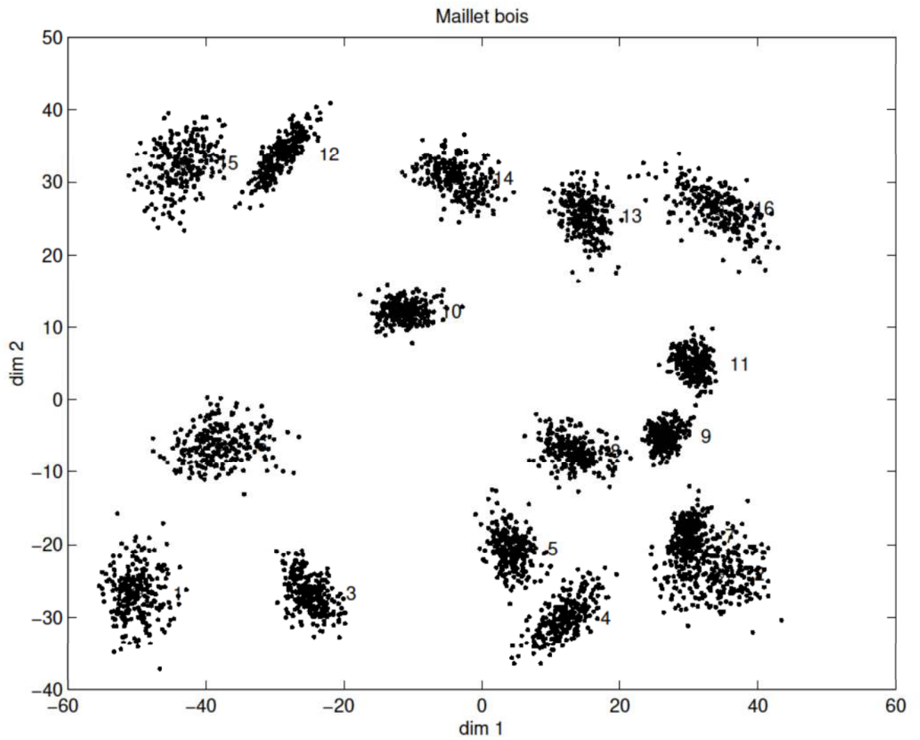
FIG. A.1 – Bootstrap : distribution des nuages sur 250 tirages, maillet bois.
