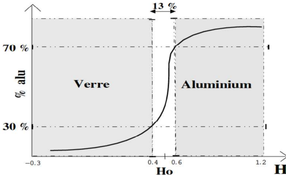
FIG. 9.10 – Représentation de la sigmoïde moyenne ajustée sur les courbes de réponses. Le changement rapide de perception du matériau montre une catégorisation des stimuli par les sujets.
