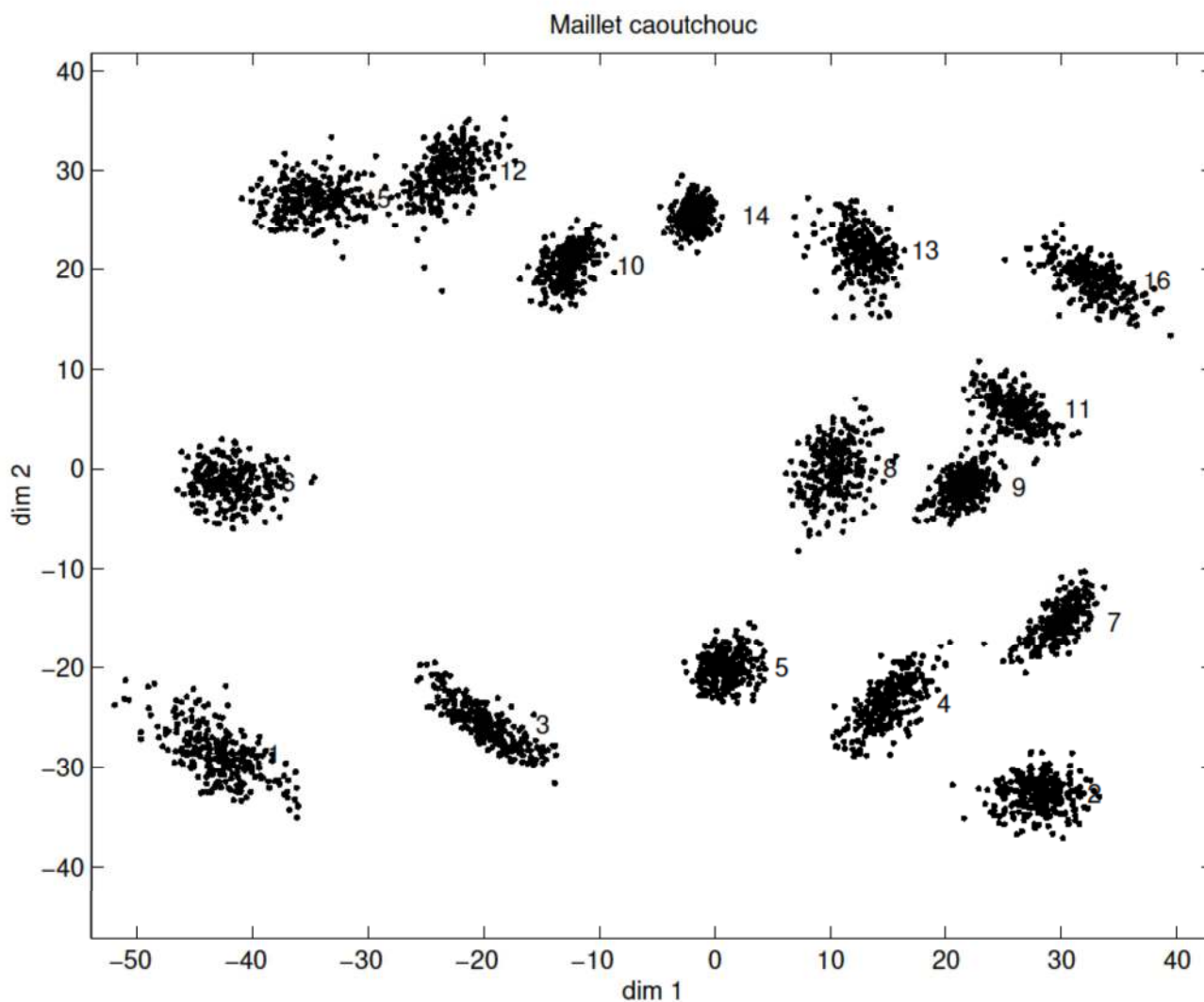
FIG. A.2 – Bootstrap : distribution des nuages sur 250 tirages, maillet caoutchouc.
