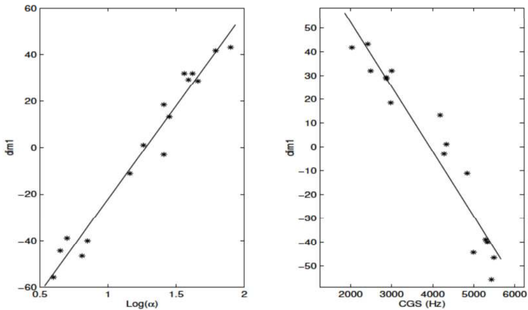
FIG. 7.6 – Représentation des corrélations entre la dimension perceptive dim1 et les paramètres analytiques ( \alpha , CGS ) séparément
