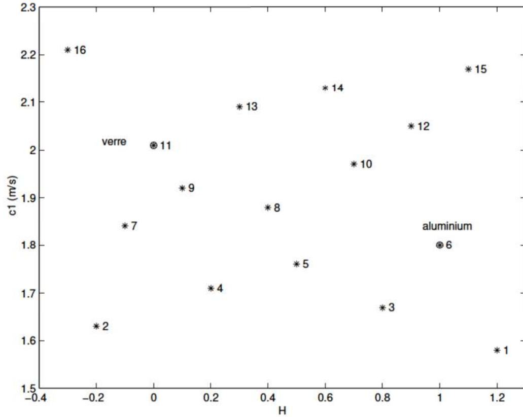
FIG. 9.2 – Représentation spatiale des stimuli dans le plan amortissement-élasticité. L'amortissement est représenté par la valeur H du coefficient d'interpolation et l'élasticité est représenté par c_1 . Les stimuli 6 et 11 correspondent aux valeurs exactes de la synthèse respectivement pour l'aluminium et le verre.
