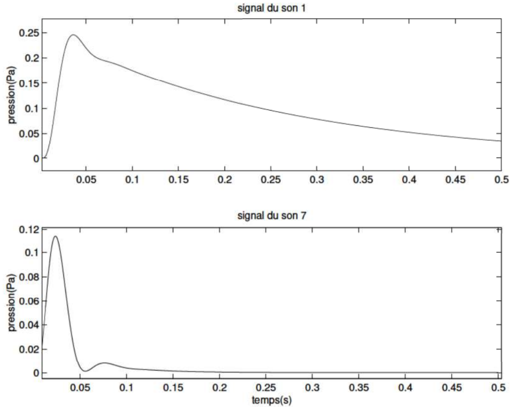
FIG. 7.3 – Evolution temporelle pour les sons 1 et 7 représentant respectivement le plus faible et le plus fort amortissement.
