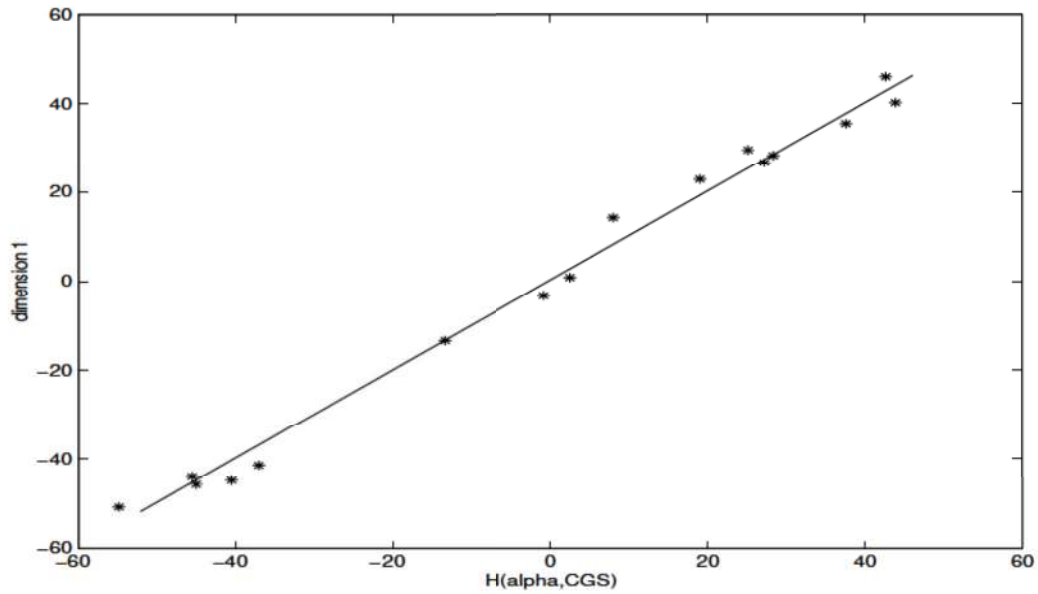
FIG. 7.7 – Régression multiple de \alpha et CGS sur la dimension perceptive dim1
