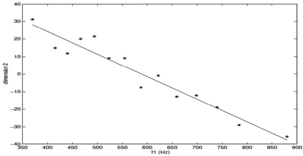
FIG. 8.6 – Représentation de la corrélation entre la dimension perceptive dim2 et la fréquence imposée au programme f_1 .
