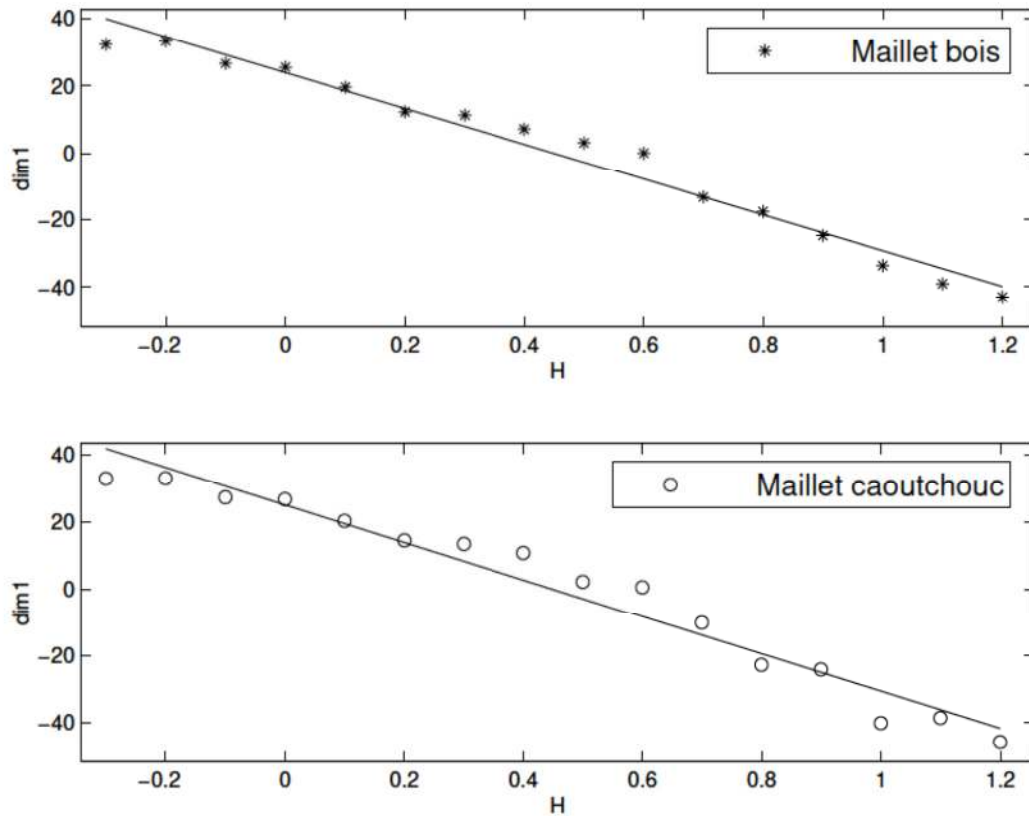
FIG. 9.9 – Corrélation entre H , coefficient d'interpolation du modèle de perte, et la dimension perceptive dim1 .
