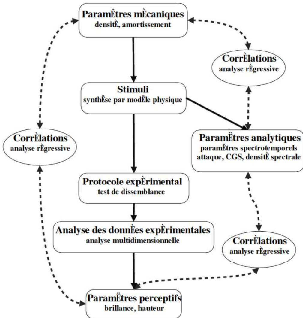
FIG. 6.1 – Les sons sont construits avec les programmes de synthèse par modèle physique puis proposés aux sujets pour une expérience de dissemblance, les dimensions révélées par l'analyse multidimensionnelle sont ensuite corrélées avec les paramètres mécaniques d'une part et les paramètres analytiques des signaux d'autre part.
