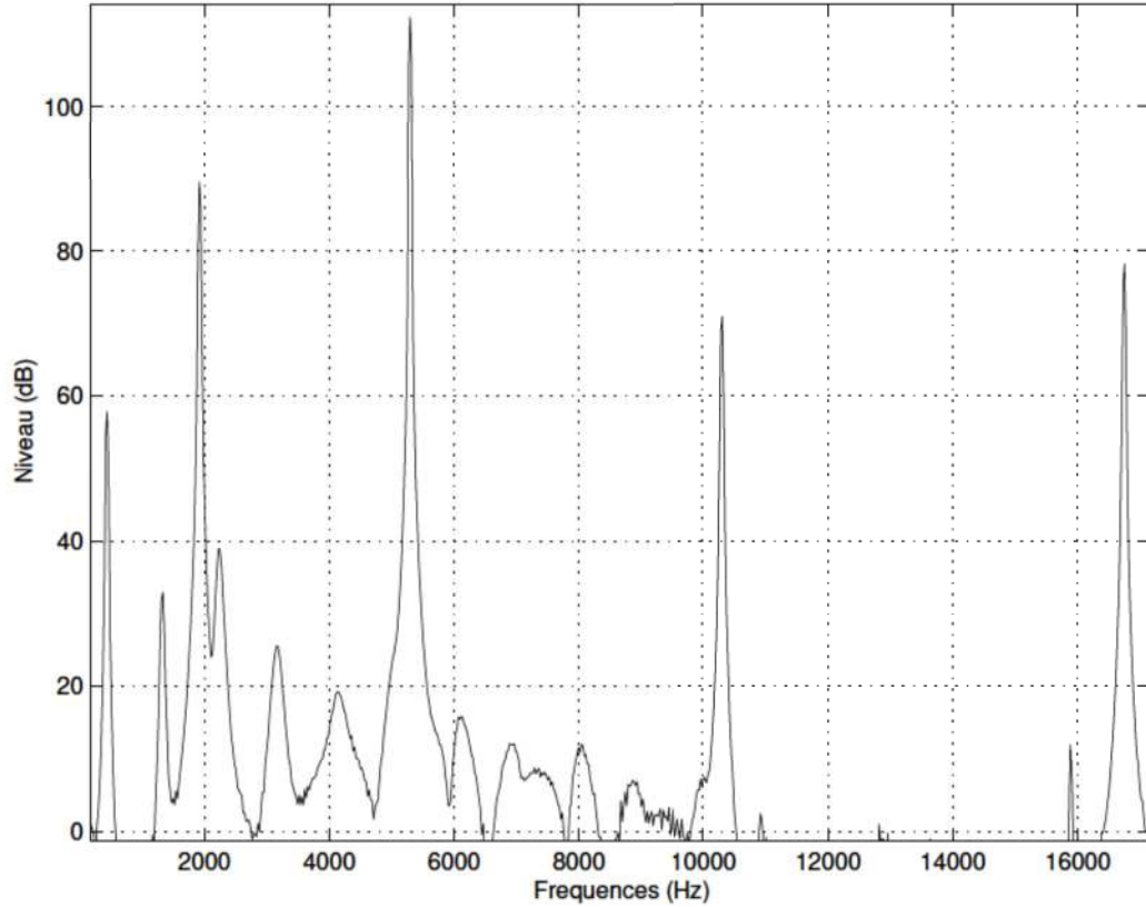
FIG. 7.2 – Spectre du son 10 calculé sur 85 \text{ ms} ( 2048 \text{ points} ) à partir de la fin de l'attaque ( 23 \text{ ms} )
