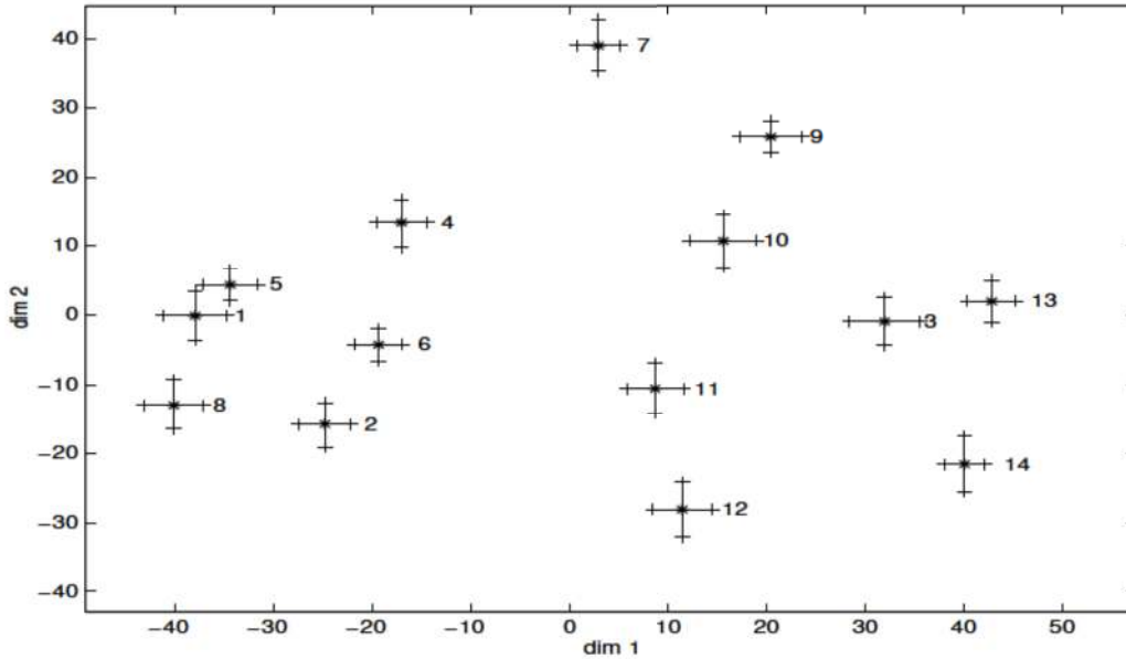
FIG. 8.3 – Espace perceptif rendu par l'analyse MDS, les écarts-types sont estimés par l'analyse bootstrap sur 250 tirages.
