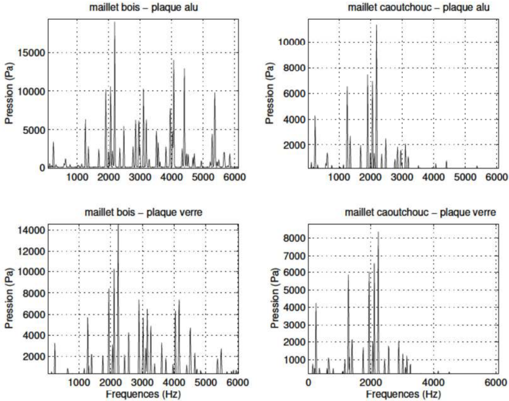
FIG. 9.3 – Représentation spectrale des plaques 6 et 11 caractéristiques de l'aluminium et du verre, frappées par des maillets en bois et en caoutchouc. Les niveaux sont alignés sur les maximums tels qu'ils sont présentés aux sujets. Les spectres ont été calculés sur une fenêtre temporelle de 22 ms à partir de 1 ms du début du son ( N = 1024 points, f_e = 48kHz ).
