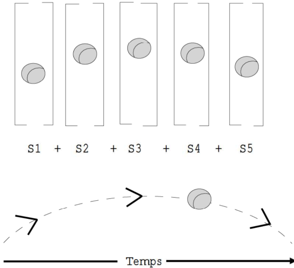
FIG. 3.1 – Représentation traditionnelle et écologique des évènements et stimuli ; la partie supérieure représente la vue traditionnelle avec décomposition de l'évènement en une suite d'instant, chacun décrit par son propre stimulus S_i ; pour percevoir l'évènement il faut rassembler les stimuli ensemble et reconstituer la dynamique. Dans la partie inférieure l'information recouvre le temps et ce dans la même durée que l'évènement. La tâche de celui qui perçoit est de détecter l'évènement spécifié par l'information (d'après Michaels et Carello [53]).
