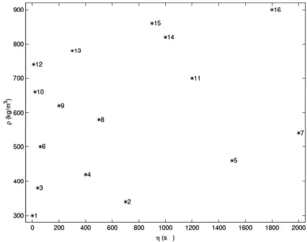
FIG. 7.1 – Représentation des sons dans l'espace physique (\eta, \rho)
