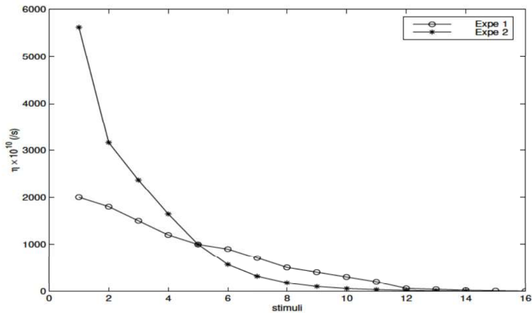
FIG. 8.1 – Choix des paramètres mécaniques. Les stimuli sont renumérotés dans l'ordre de l'amortissement décroissant.
