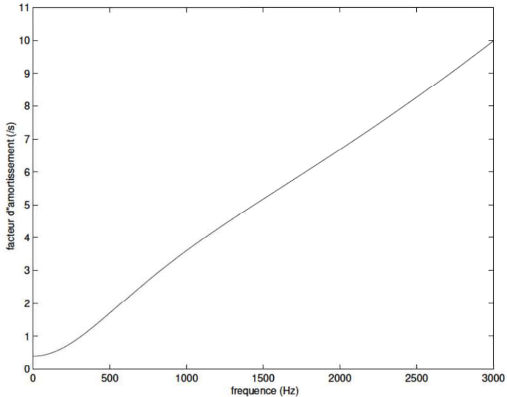
FIG. 9.1 – Courbe représentant le facteur d'amortissement théorique calculé sur le modèle de pertes viscoélastiques en fonction de la fréquence.
