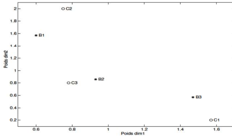
FIG. 9.6 – Espace des poids pour chaque classe sur les dimensions 1 et 2 ( C =caoutchouc, B =bois).
