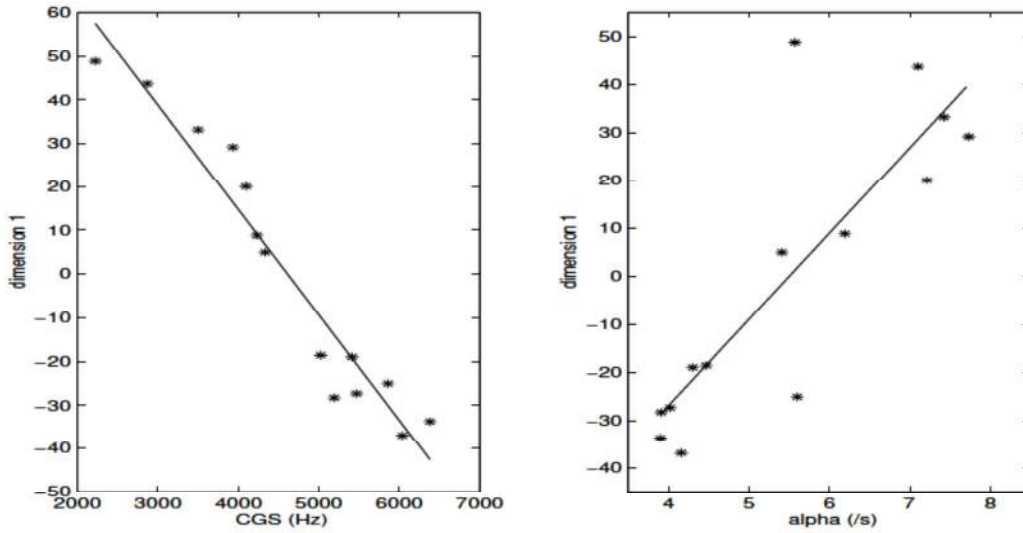
FIG. 8.4 – Représentation de la corrélation entre la dimension perceptive dim1 et la régression multiple sur les deux paramètres analytiques CGS et \alpha .
