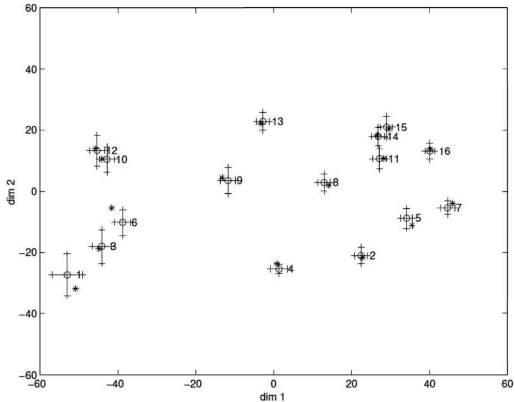
FIG. 7.4 – Représentation des sons dans l'espace perceptif. La dimension 1 représente le timbre et la dimension 2 la hauteur des sons. Les écarts-types ont été calculés à partir d'une analyse bootstrap sur 250 tirages. Les * symbolisent les résultats de CLASCAL, les o représentent les valeurs moyennes après calcul par bootstrap
