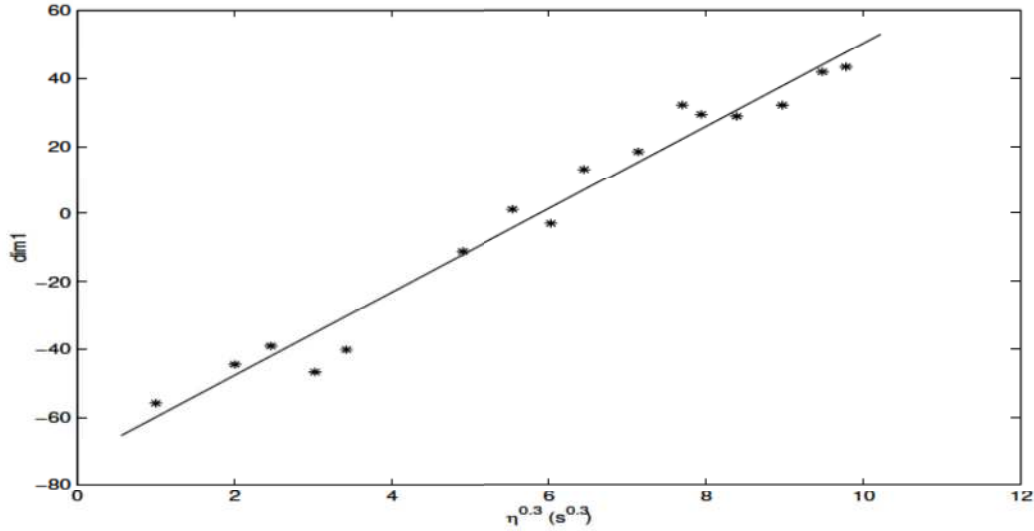
FIG. 7.9 – Représentation de la corrélation entre la dimension perceptive dim1 et le paramètre d'amortissement \eta
