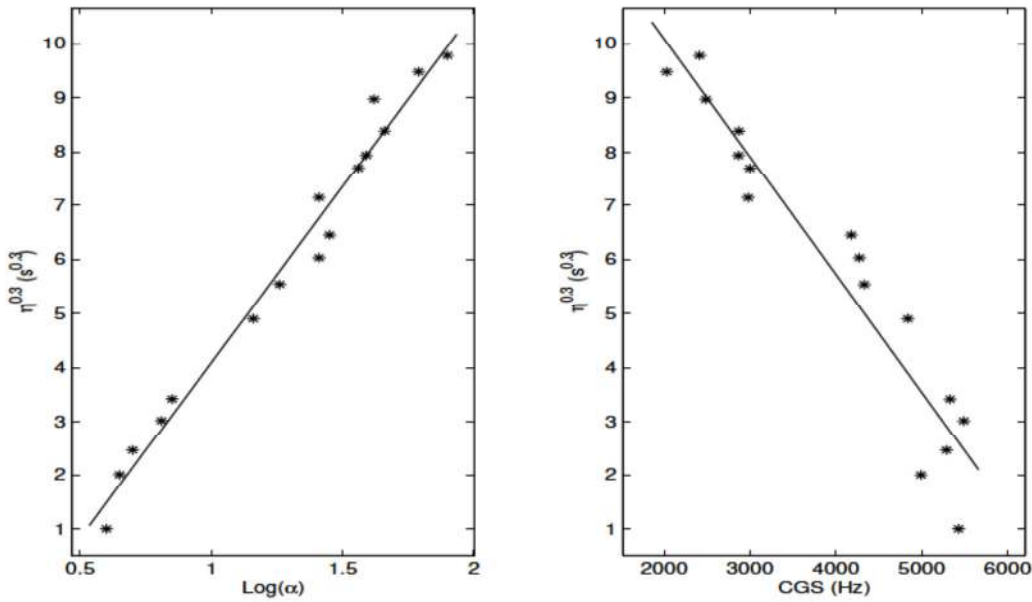
FIG. 7.8 – Représentation des corrélations entre le terme d’amortissement \eta et les paramètres analytiques ( \alpha , CGS).
