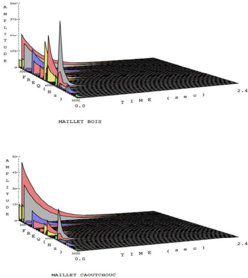
FIG. 9.5 – Visualisation 3D de la gamme de fréquences [3000 – 5000 Hz]. Les modes excités par les plaques frappées avec le maillet dur (bois) sont moins amortis que ceux excités par le maillet caoutchouc. Les niveaux sont ajustés sur le maximum d'amplitude de la gamme de fréquence, les stimuli étant égalisés eux-mêmes en sonie avant l'expérience.
