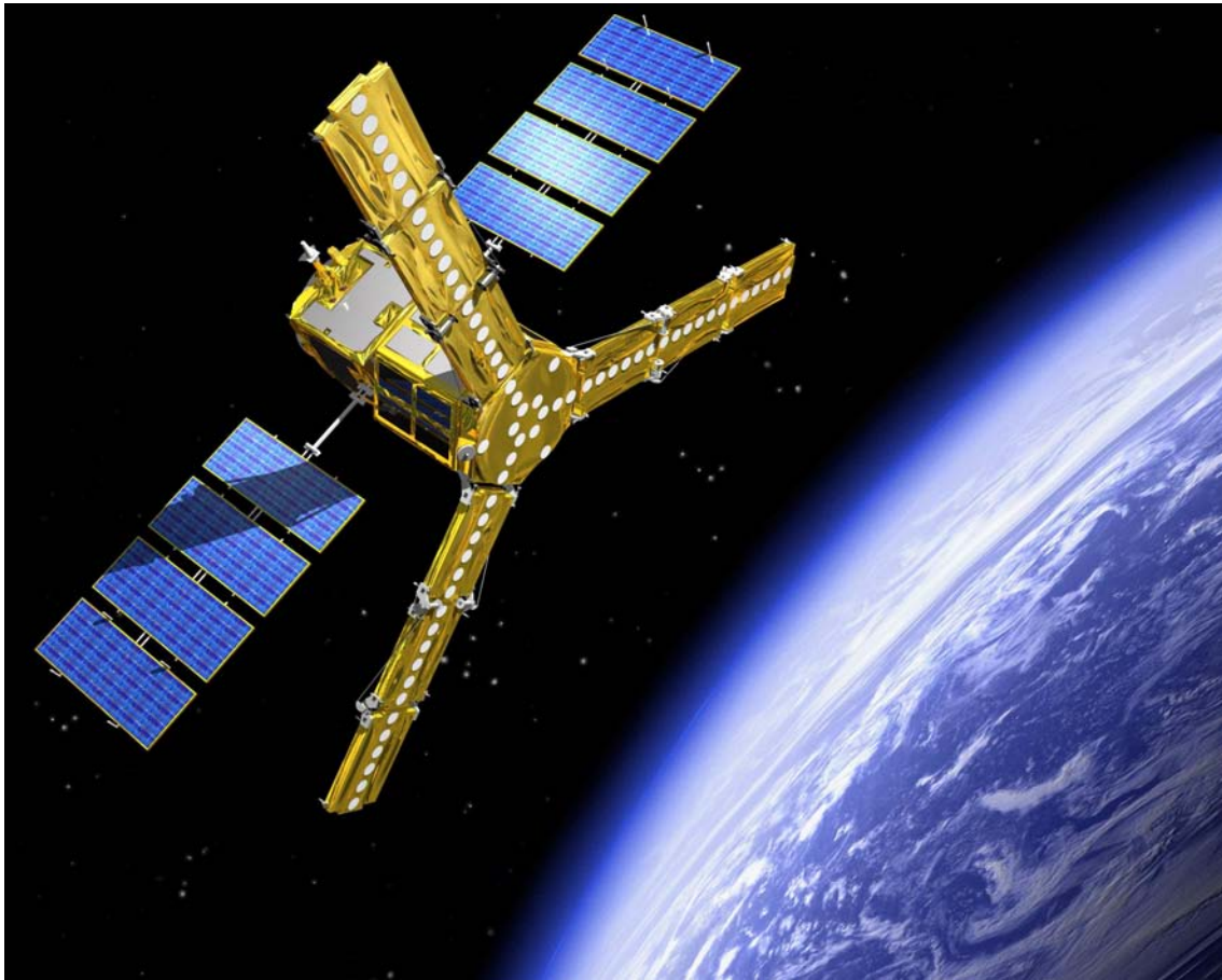
FIG. 1.6 – Satellite SMOS : vue de l'artiste.
