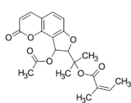
isoedultin
