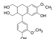
cyclolariciresinol
