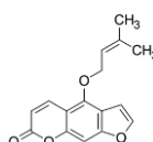
isoimperatorin
