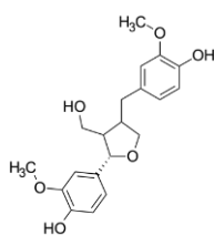
lariciresinol
