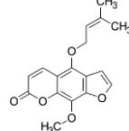
cnidiin
