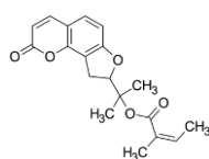
columbianadin
