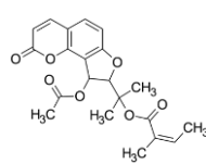
isoedultin
