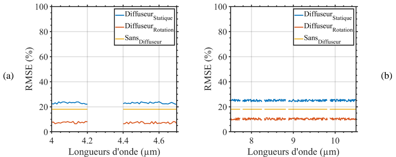
Figure 35 : Les graphes présentant les résultats du RMSE pour les deux caméras (a) SC5000 et (b) A65 suivant les différentes longueurs d'onde.
