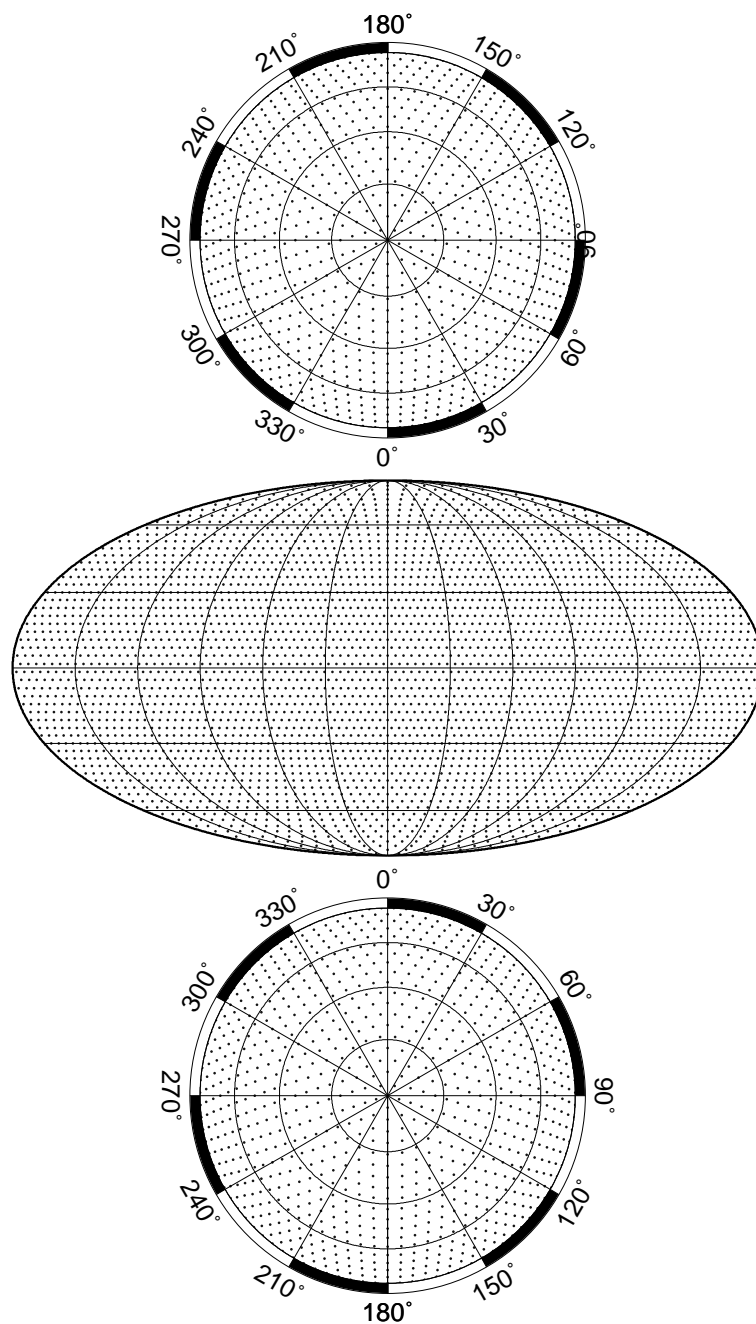
FIG. 7.1 – Distribution icosaédrale de dipôles (vue du pôle nord, projection Molweide et vue du pôle sud). Le paramètre de bande est égal à 20, soit 3612 dipôles avec un espacement moyen de 3,4^\circ .
