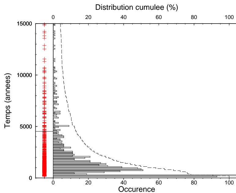
FIG. 3.8 – Distribution des temps aléatoires pour la tache 3 (“+”). Le temps vrai (tableau 3.4) est indiqué par un trait horizontal, et la distribution cumulée des temps est tracée en pointillés.
