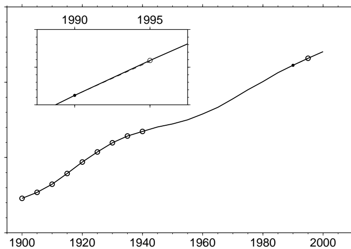
FIG. 2.8 – 7 ème génération de l'IGRF : Adoption des IGRF 1900 à 1940 et 1995, et du DGRF 1990. La variation séculaire de l'IGRF 1990 est exacte à 3%.
