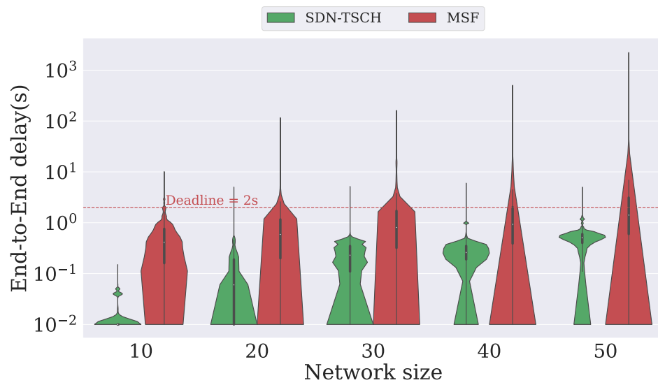
Figure 6: Latence de bout en bout
