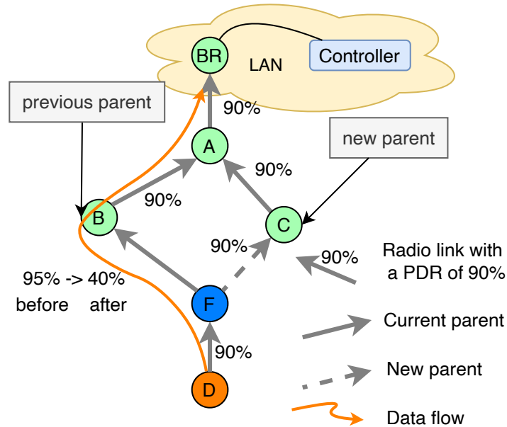
Figure 8: Un contrôleur doit reconfigurer les plans de contrôle et de données pour rediriger les flux à travers le lien ( F \rightarrow C ) lorsque le PDR du lien ( F \rightarrow B ) diminue de 95% à 40%
