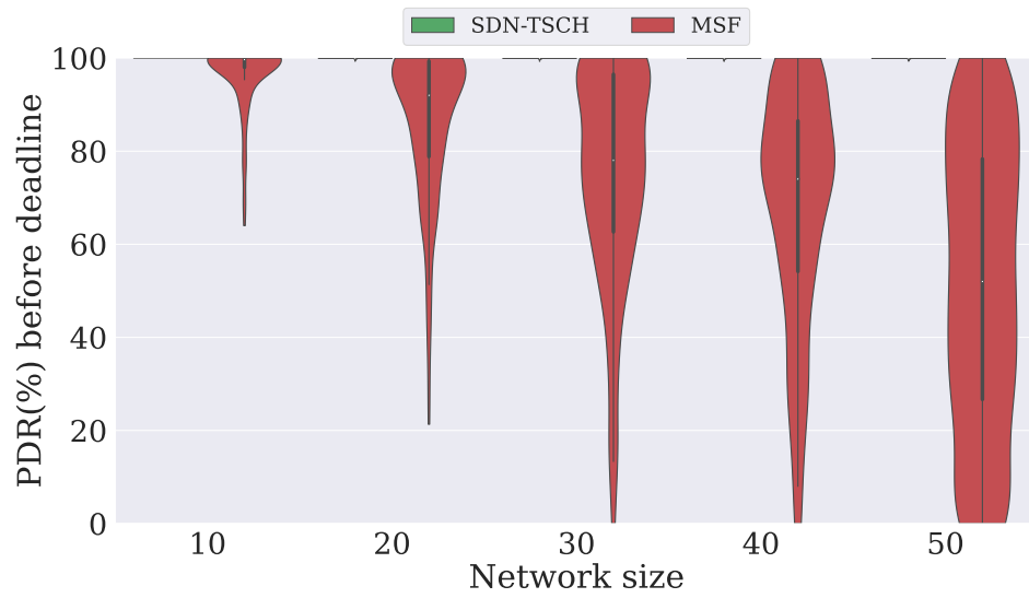
Figure 5: Taux de remise de paquets (PDR) des flux avant la date limite
