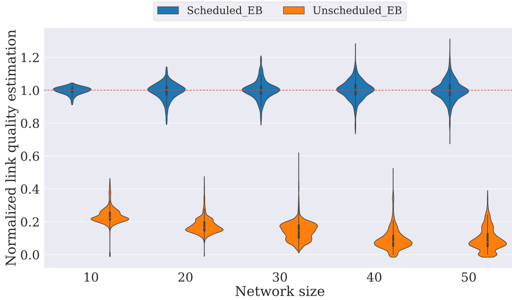
Figure 7: Estimation de la qualité de liaison
