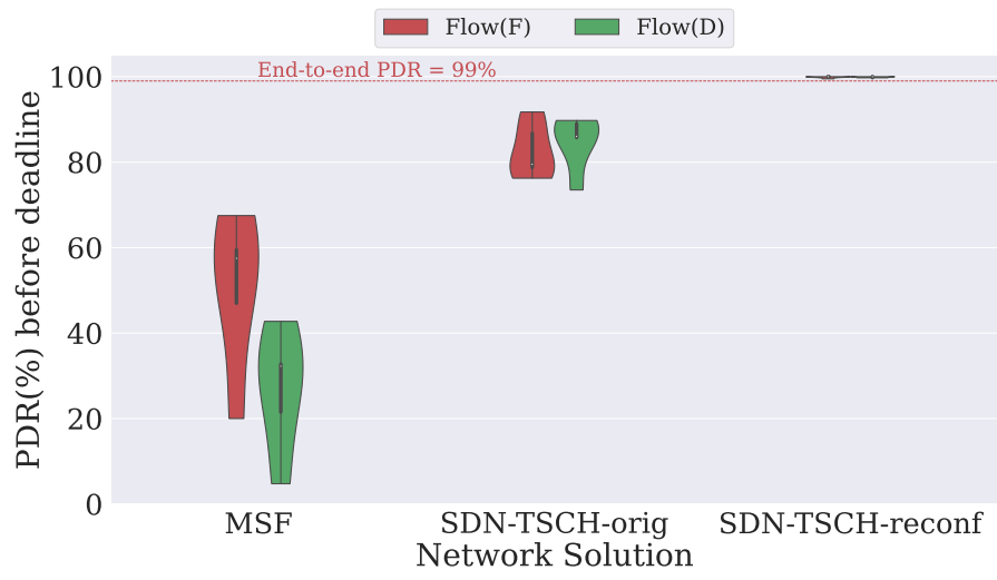
Figure 9: Taux de Livraison de Paquets par Flux
