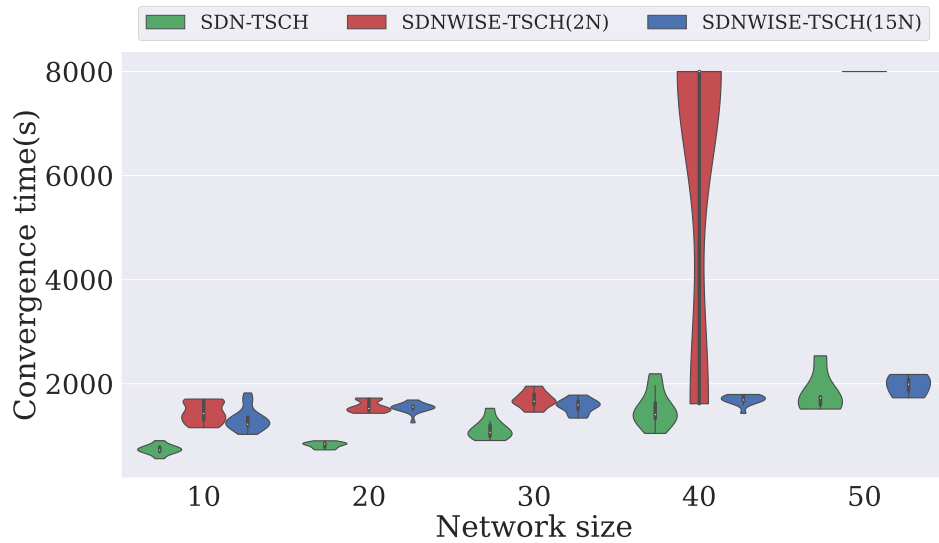
Figure 3: Temps de convergence du réseau
