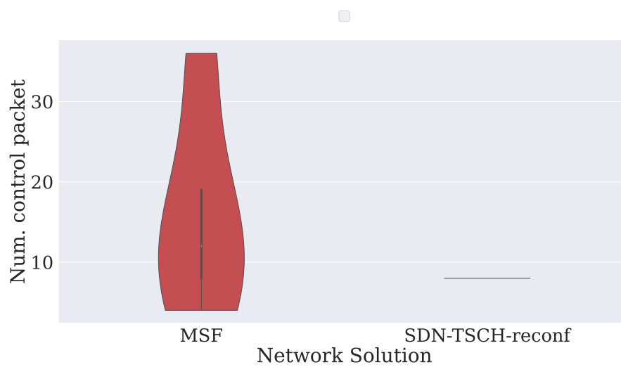
Figure 11: Surcharge de Contrôle pour la Reconfiguration
