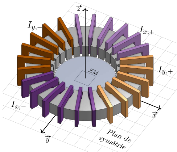
(a) Vue de la simulation 3D (avec ZM la zone de mesure de 20\text{ mm} \times 20\text{ mm} ).
