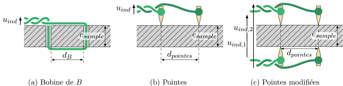
FIGURE 2.10 – Différentes méthodes de mesure de l'induction magnétique B sous la forme d'une ou plusieurs tensions induites u_{ind,i} .
