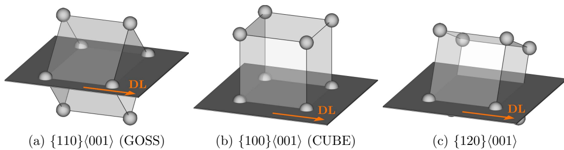
FIGURE 1.6 – Les principales textures spécifiques développées, exprimées sous la forme \{\text{Plan de la tôle}\}\langle \text{Direction de laminage} \rangle . Les mailles représentées ici sont cubiques, mais pourraient être centrées ou faces centrées.
