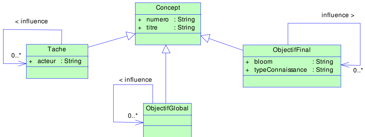
Figure 4-8 : représentation UML des dépendances du modèle de contenus
