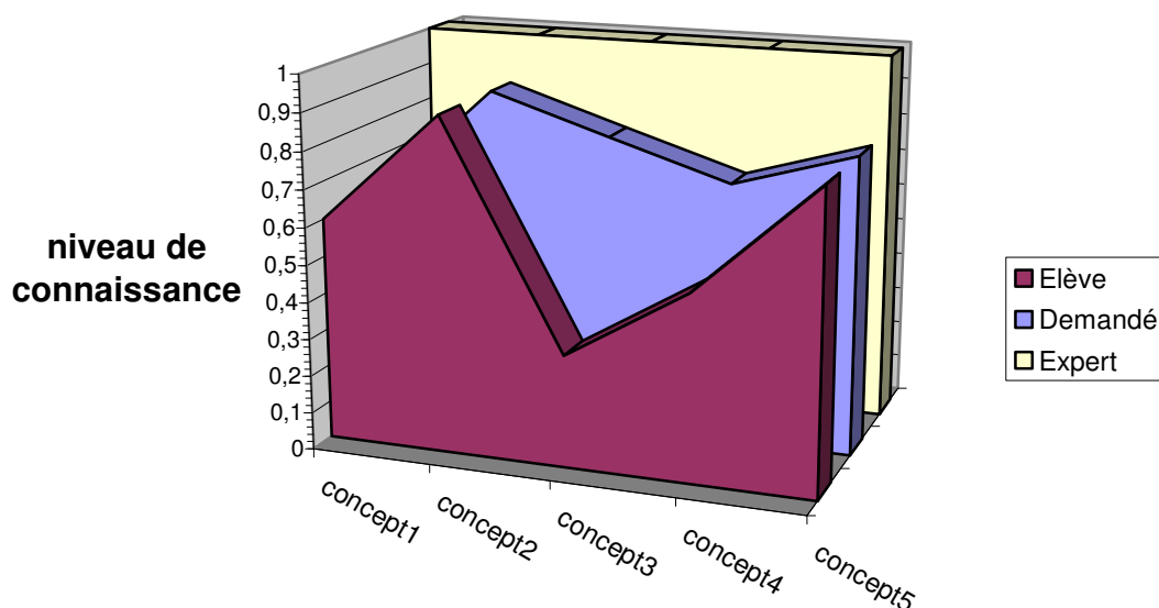
Figure 1-3 : Modèle différentiel
