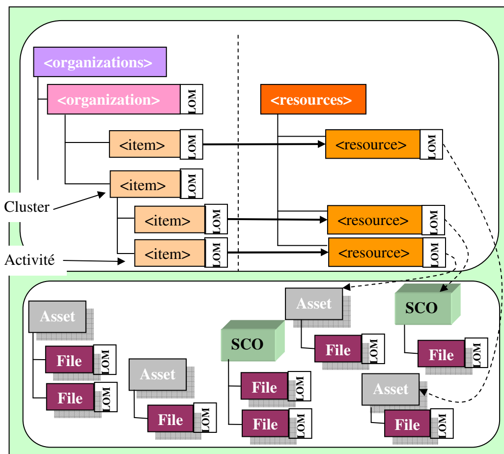
Figure 4-13 : métadonnées LOM
