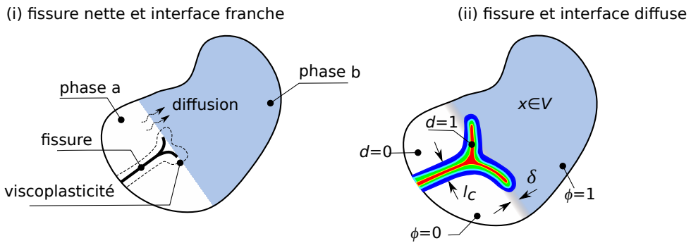
(b) Régularisation des singularités mobiles (fissuration, oxydation) par des approches champ de phase, les fronts sont diffus représentés par une variable d'endommagement d évoluant de façon continue sur une longueur l_c pour la fissuration, et par une variable d'ordre \phi évoluant de façon continue sur une longueur \delta pour l'oxydation. Représentation du problème avec singularités (a) non régularisées, (b) régularisées.
