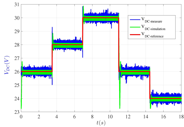
FIGURE 3.36 – Variation de la référence de tension de bus continu pour vitesse égale à 800 tr/mn et une charge de 15 Ohm
