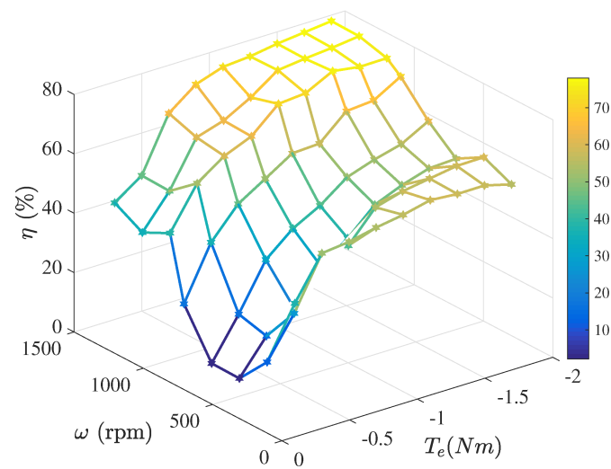
FIGURE 3.39 – Cartographie de rendement expérimentale[75]
