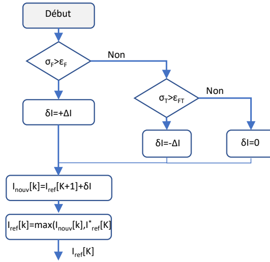
FIGURE 3.10 – Adaptateur du courant.
