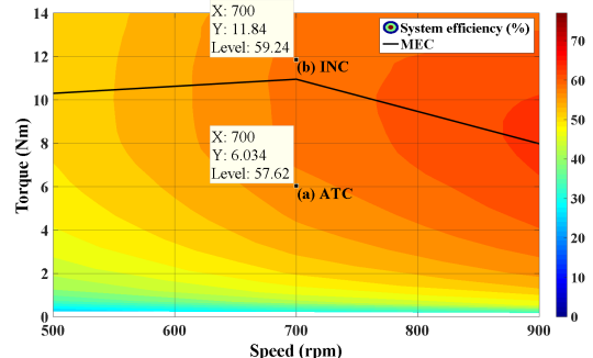
FIGURE 3.25 – zoom de cartographie de rendement avec l'ATC
