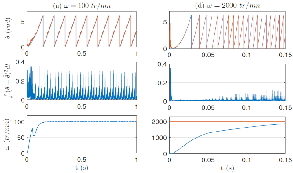
FIGURE 4.9 – Résultats de l'estimation de la position avec la méthode de flux M2
