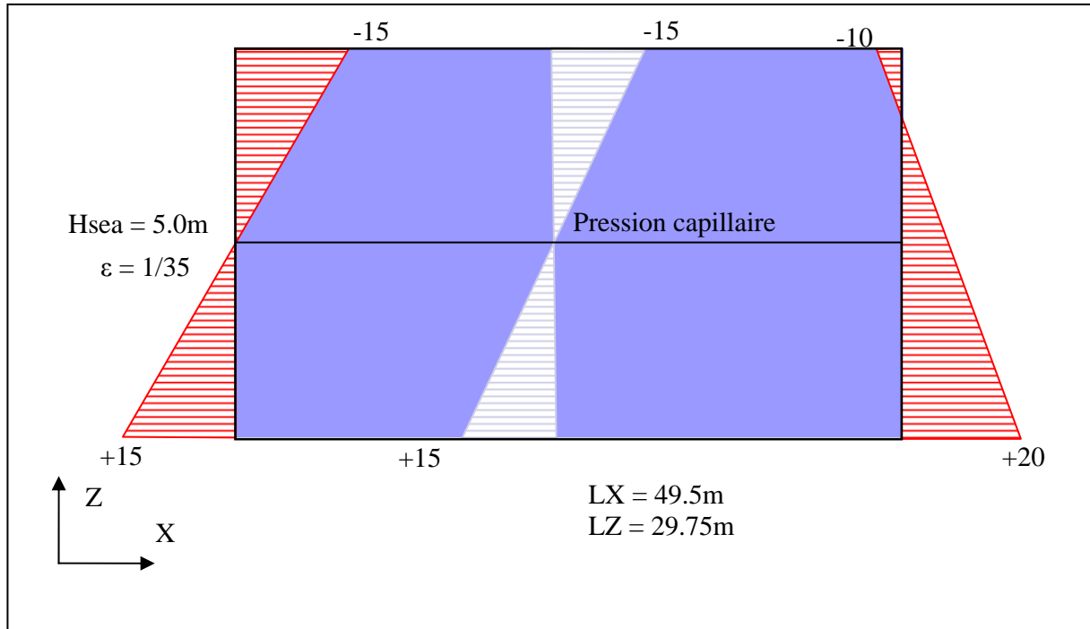
Fig. 3.11 Configuration du problème de Glover pour le cas test.
