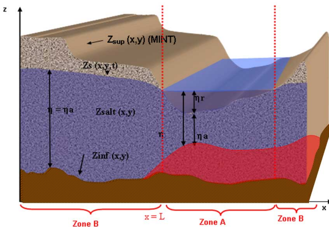
Fig. 5.2. Représentation schématique d'un modèle des écoulements plans bicouche avec intrusion saline (vu ici en perspective).
