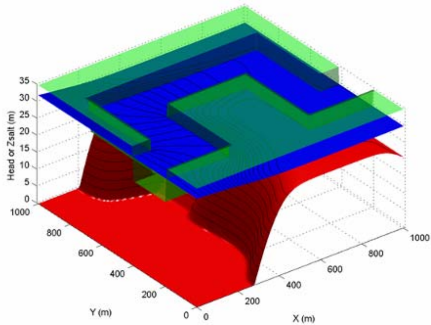
Fig. 5.9. Simulation transitoire simplifiée rivière/aquifère en présence d'intrusion saline avec le model couplé 2D plan de BIGFLOW (méandre rectangulaire sans pente) ( t=45s ).
