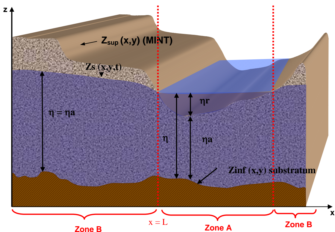
Fig. 5.1 Représentation schématique en perspective d'un modèle d'écoulement plan à deux couches. (Voir la section V.3.2 pour la description des variables).
