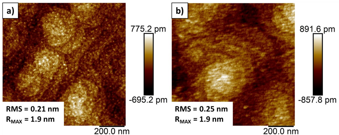
Figure III.35 : Mesures AFM 1 \times 1 \mu\text{m} de la surface de AlGaN pour l'échantillon après une gravure au plasma (a) \text{SF}_6/\text{Ar} , et (b) \text{CHF}_3/\text{CF}_4/\text{Ar} à basse énergie ionique avec 200 % du temps de sur-gravure appliqué.
