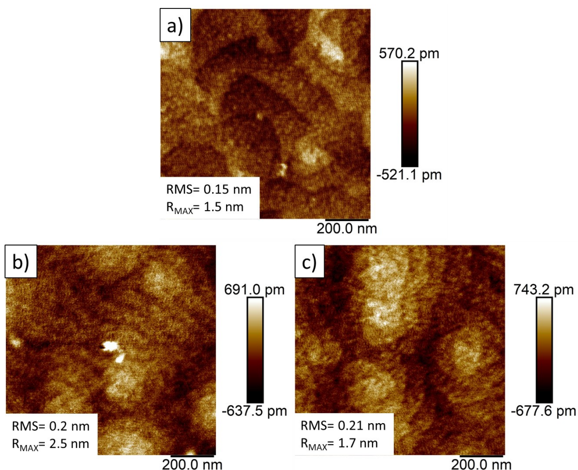
Figure III.16 : Mesures AFM de la surface de AlGa N pour (a) l'échantillon de référence et pour l'échantillon après une gravure au plasma (b) SF 6 /Ar et (c) CHF 3 /CF 4 /Ar à haute énergie ionique (260 eV).
