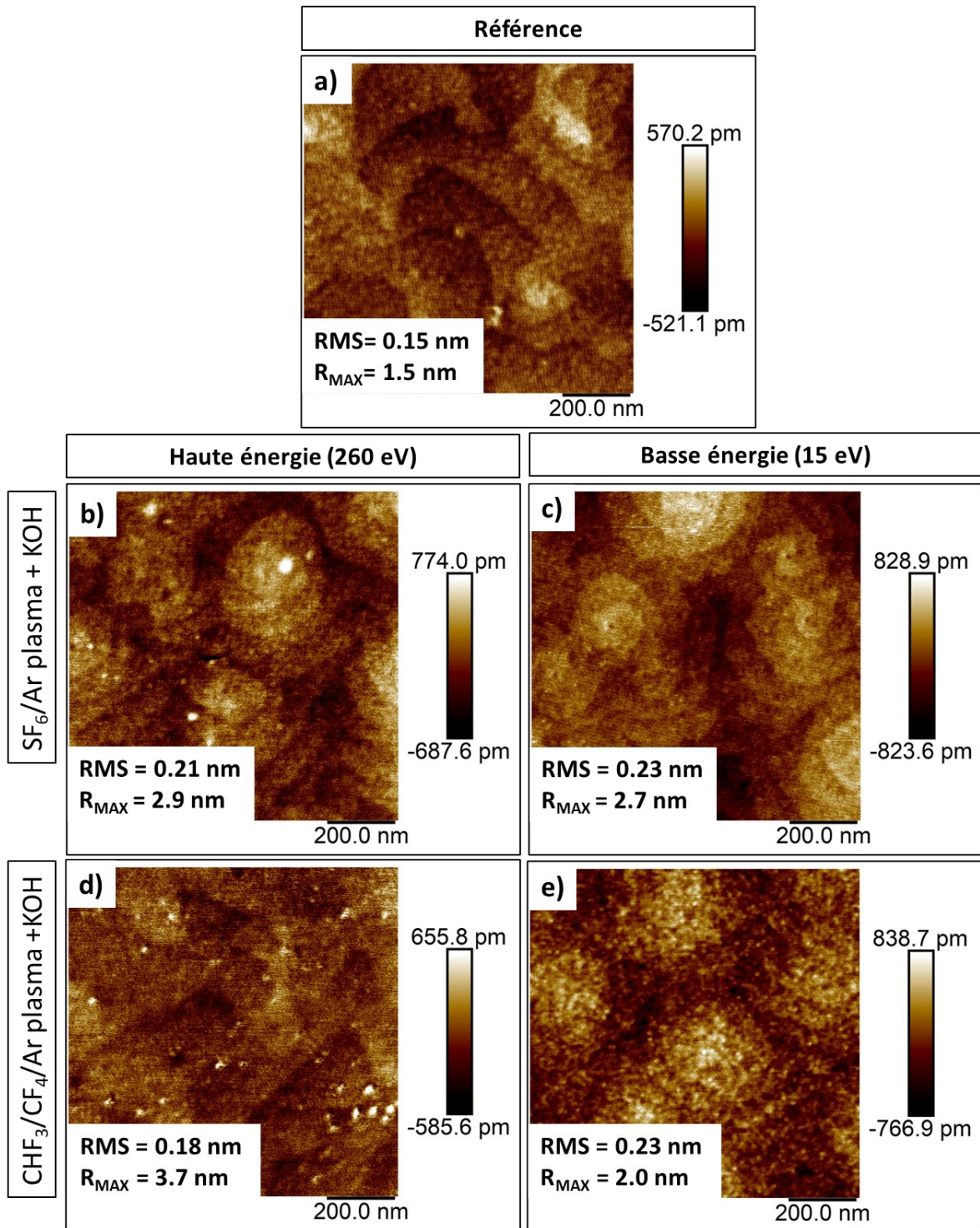
Figure V.9 : Mesures AFM de la surface de la couche AlGaN pour les échantillons (a) référence et après gravure par plasma (b) SF 6 /Ar et (c) CHF 3 /CF 4 /Ar à haute énergie ionique (260 eV); et après gravure au plasma (d) SF 6 /Ar et (e) CHF 3 /CF 4 /Ar à basse énergie ionique (15 eV) suivie d'un traitement KOH.
