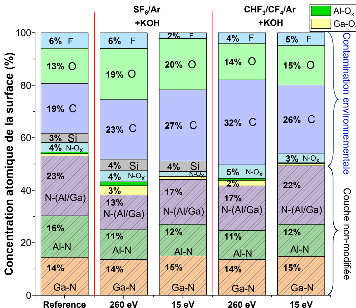
Figure V.2 : Composition chimique de la surface de la couche AlGaN à l'angle de 76,25° (surface) pour l'échantillon de référence (gravure du SiN par BOE) et les échantillons après gravure du SiN par le plasma SF 6 /Ar et CHF 3 /CF 4 /Ar à haute et basse énergie ionique (260 et 15 eV) suivie par l'étape de nettoyage KOH.
