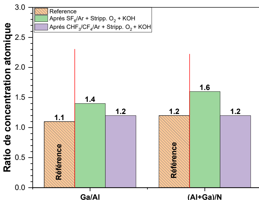
Figure V.6 : Les ratios stœchiométriques Al/Ga et (Al+Ga)/N de la surface AlGaIn à l'angle rasant de 76,25° (surface) après gravure de la passivation SiN par le SF 6 /Ar et CHF 3 /CF 4 /Ar plasma à basse énergie ionique (15 eV) suivie par l'étape de stripping O 2 suivie par l'étape de nettoyage KOH.
