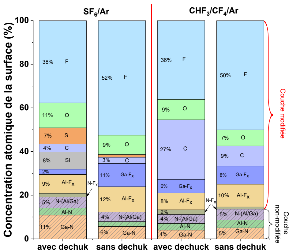
Figure III.11 : Composition chimique de la surface des échantillons de AlGaN à l'angle de 76,75° (surface) après la gravure du SiN par le plasma SF 6 /Ar et CHF 3 /CF 4 /Ar à haute énergie ionique en fonction d'utilisation de dechuck .
