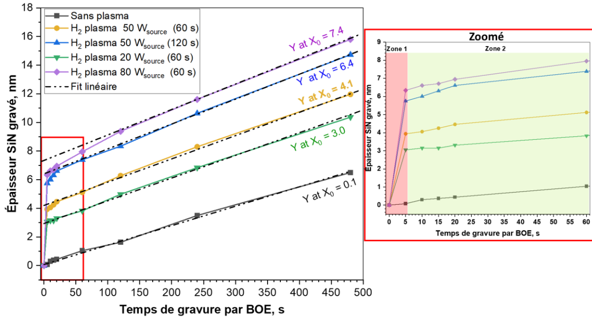
Figure IV.6 : Épaisseur de SiN gravée en fonction de la durée du bain BOE pour l'échantillon non exposé au plasma, ainsi que pour les échantillons exposés à un plasma CCP d' H_2 avec différentes conditions.
