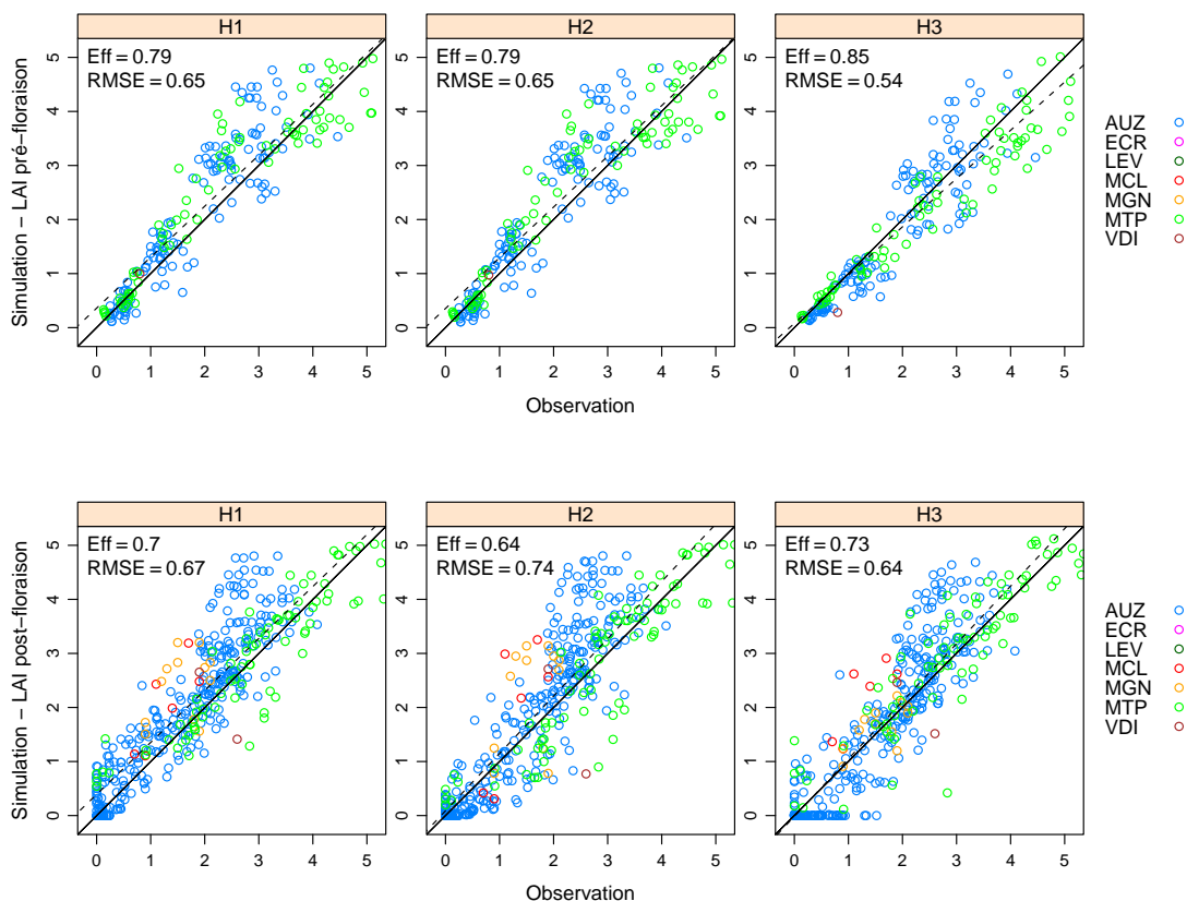
FIG. 6.2: Evaluation des trois hypothèses de modélisation pour la phase d'expansion de la surface foliaire (haut) et pour la phase de sénescence (bas).
