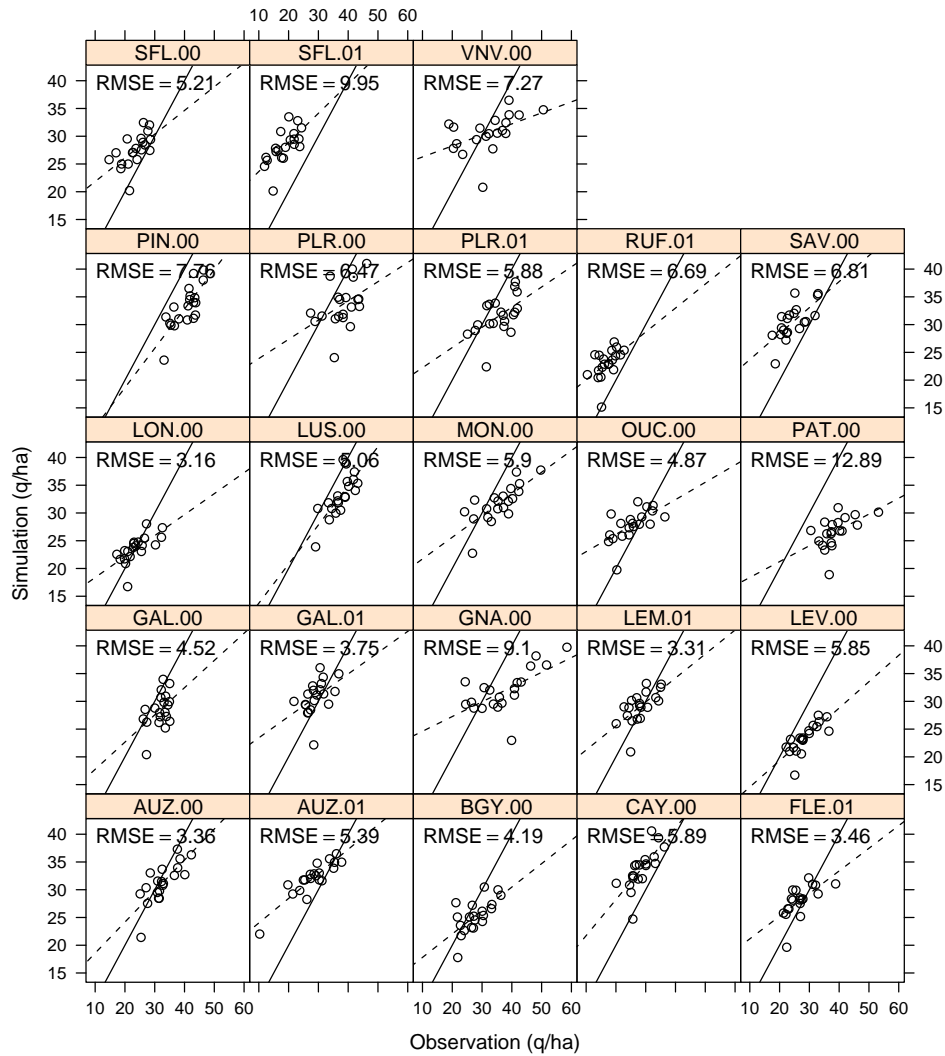
FIG. 10.3: Rendement simulé en fonction du rendement observé pour 20 géotypes présents sur 23 situations (site x année) d'un réseau d'essais. La ligne pleine indique la première bissectrice, celle en pointillé est la droite de régression.
