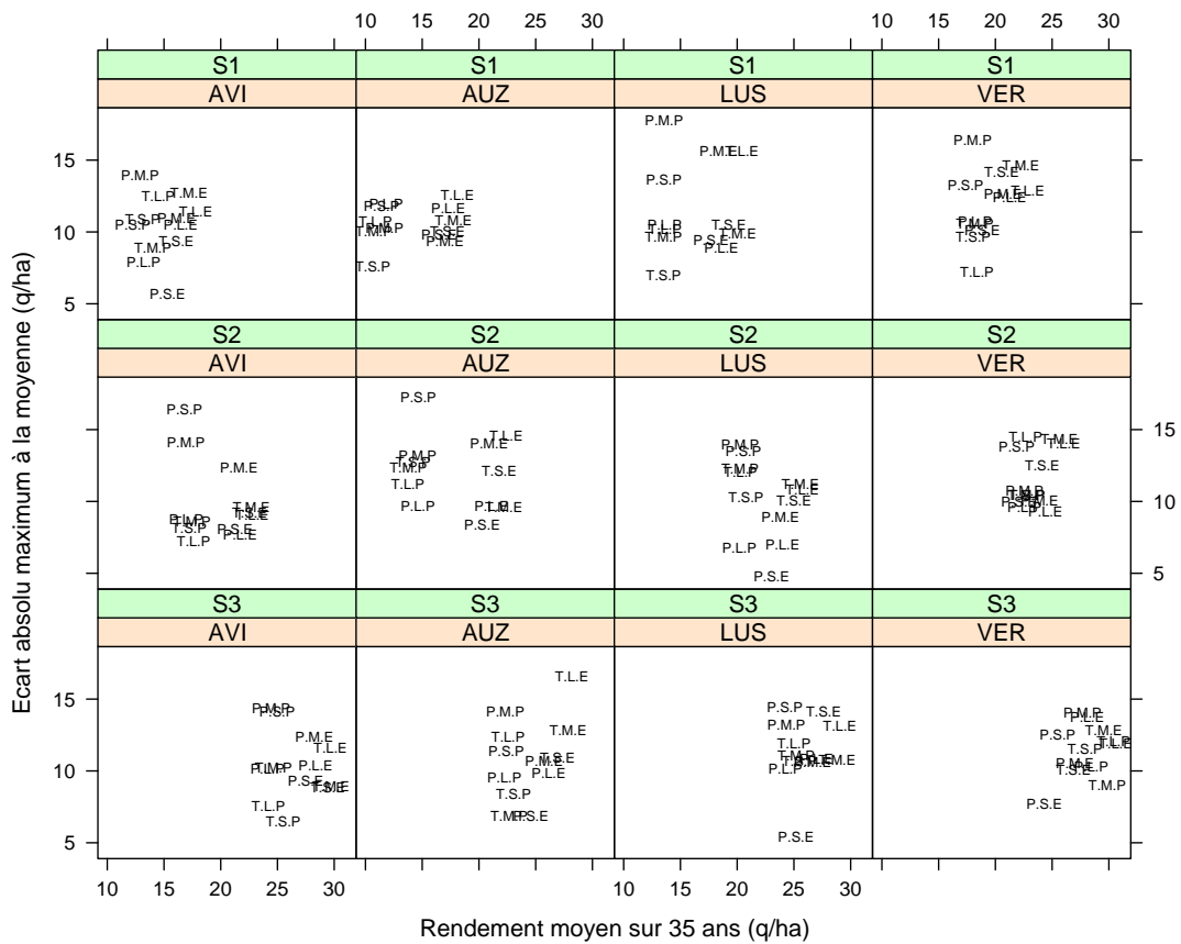
FIG. 13.9: Risque maximum d'un écart de performance selon la performance moyenne des 12 variétés virtuelles. Le risque est évalué par le maximum de la valeur absolue de l'écart entre la performance de la variété une année donnée et sa moyenne sur la série climatique.
