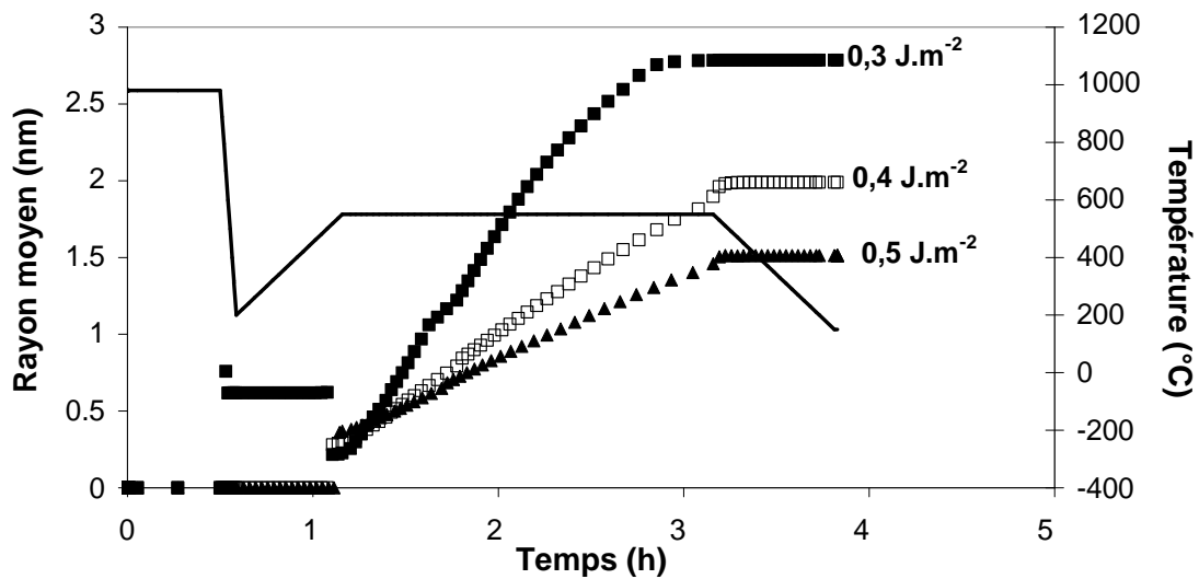
Figure III.16 : Evolution du rayon moyen des carbures M_7C_3 en fonction de l'énergie d'interface.
