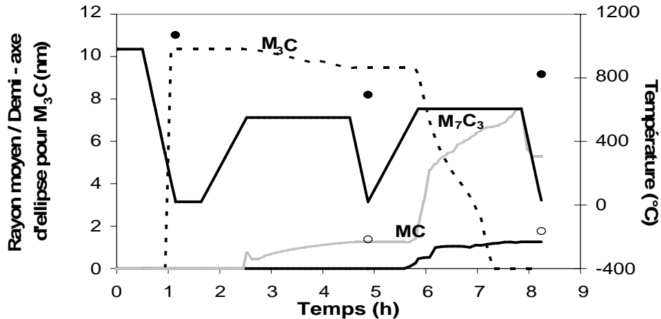
Figure III.35: Evolution des tailles des précipités au cours du traitement thermique de la nuance Co. Résultat de la méthode d'ajustement. Valeurs expérimentales issues de la DNPA des populations 1 (○) et 2 (●).
