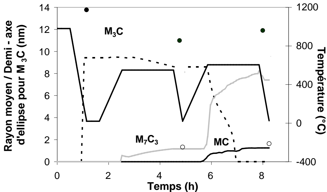
Figure III.17 : Evolution des tailles des précipités au cours du traitement thermique de la nuance X38CrMoV5. Résultat de la méthode d'ajustement. Valeurs expérimentales issues de la DNPA des populations 1 (○) et 2 (●).
