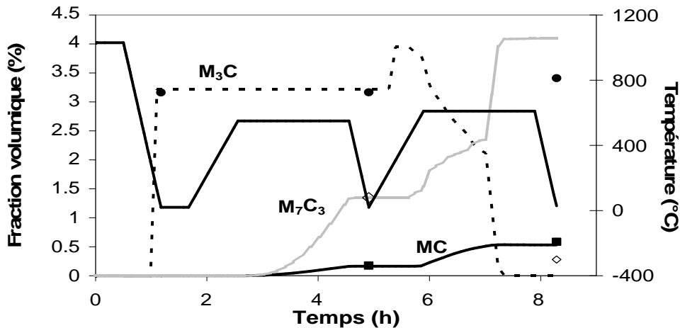
Figure III.33: Evolution des fractions volumiques des carbures au cours du traitement thermique de la nuance NiMoV. Valeurs expérimentales issues de la DNPA de la population 2 (●), des carbures Cr_7C_3 (◇) et VC (◇).
