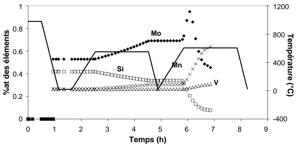
Figure III.22 : Evolutions de la composition chimique des carbures M_5C en molybdène, vanadium, silicium et manganèse au cours du traitement thermique de la nuance X38CrMoV5.
