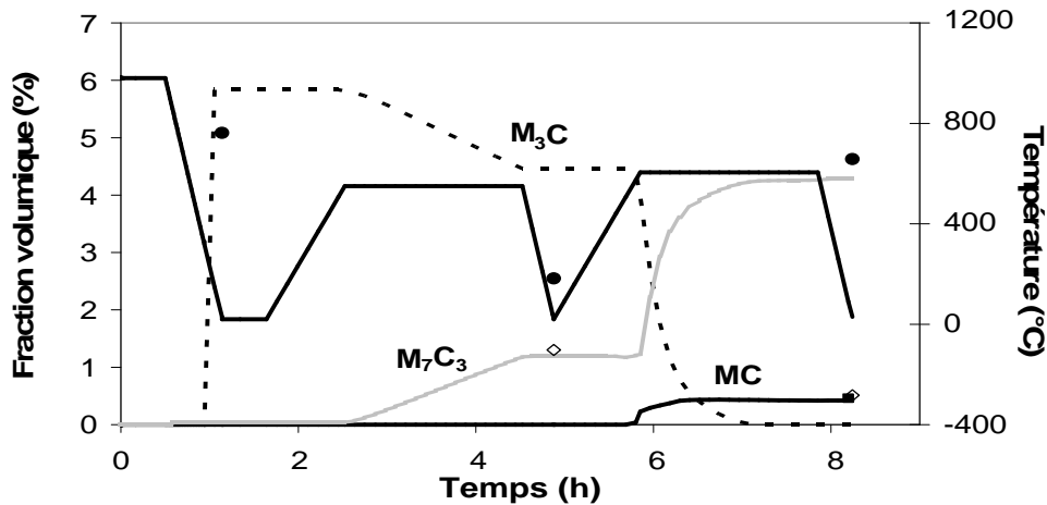
Figure III.36 : Evolution des fractions volumiques des carbures au cours du traitement thermique de la nuance Co. Valeurs expérimentales issues de la DNPA de la population 2 (●), des carbures Cr_7C_3 (◇) et VC (|).
