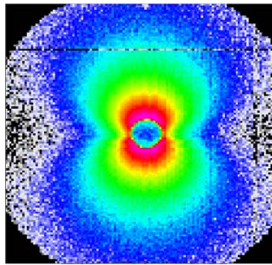
Figure I.9 : Spectre brut obtenu en DNPA en présence d'un champ magnétique saturant.
