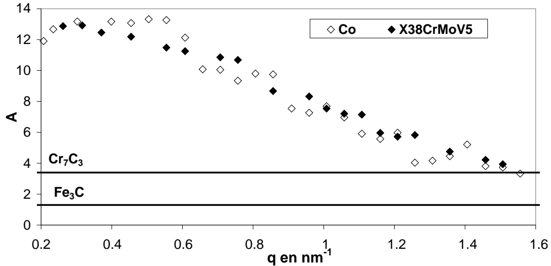
Figure II.31 : Evolution du rapport A en fonction de q des nuances X38CrMoV5 et Co trempées à l'air.
