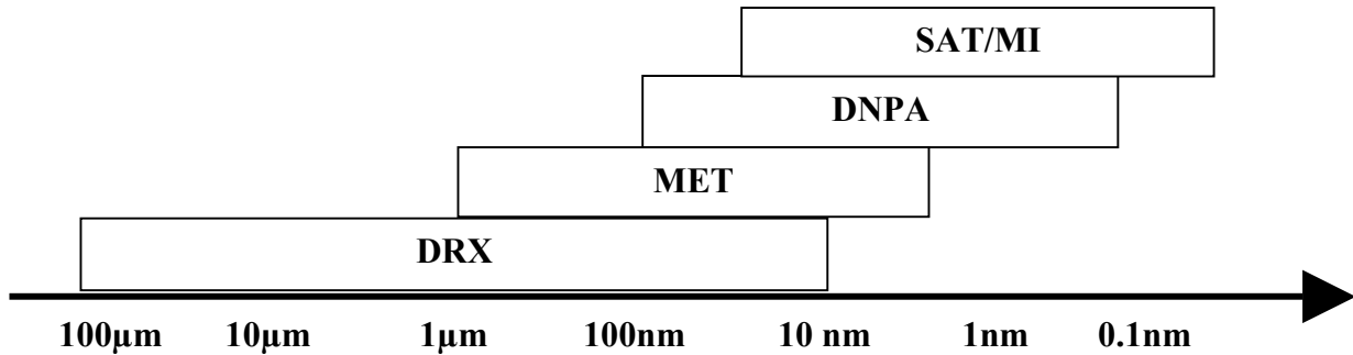
Figure I.13 : Echelles de caractérisation pour chaque technique d'investigation utilisée.
