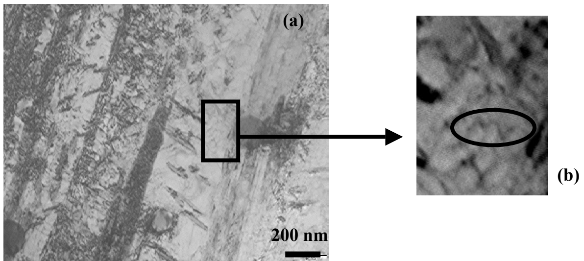
Figure II.4 : (a) Précipités allongés au sein des lattes de martensite, (b) Ancrage de dislocations sur des petits précipités.
