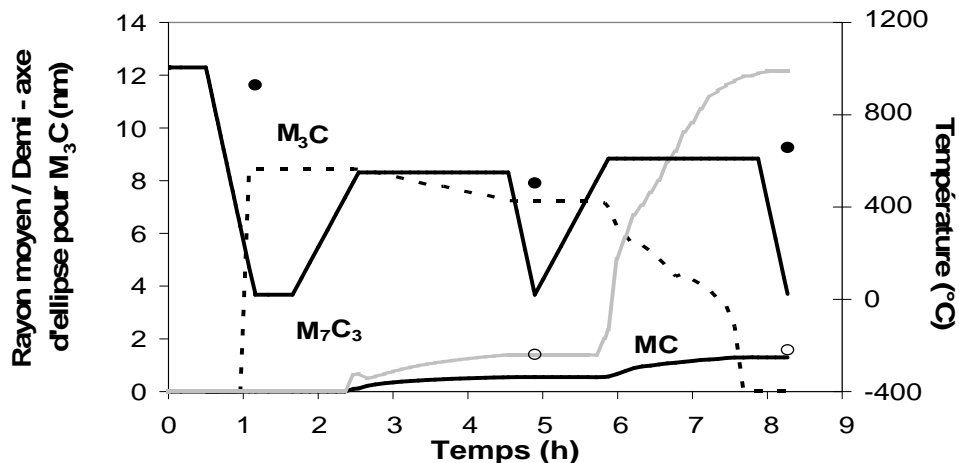
Figure III.29 : Evolution des tailles des précipités au cours du traitement thermique de la nuance Mo. Résultat de la méthode d'ajustement. Valeurs expérimentales issues de la DNPA des populations 1 (○) et 2 (●).
