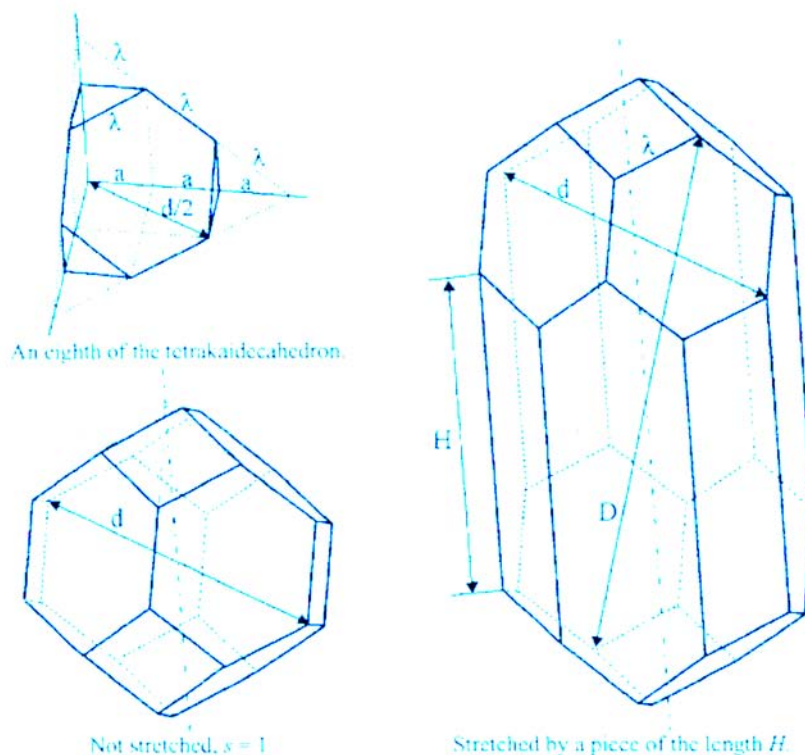
FIG. B.1: Dessin du "cube-octaèdre" utilisé dans MatCalc pour calculer le nombre de sites de germination. Construction du polyhédre, version originale et version étirée [84].
