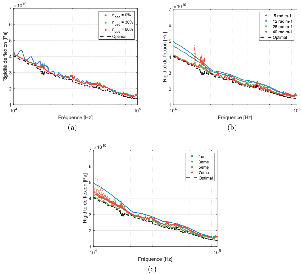
FIGURE 3.13 – Rigidité de flexion en fonction de la fréquence en faisant varier (a) le padding avec une largeur de fenêtre de 25 rad.m -1 et d'ordre 5 (b) la largeur de la fenêtre avec un zero-padding de 85% et un ordre de 5 et (c) l'ordre de la fenêtre avec un zero-padding de 85% et d'une largeur de fenêtre de 25 rad.m -1 . Ces calculs ont été réalisés sans le border-padding obtenu à partir des données expérimentales présenté à la Figure 3.12. À chaque figure est ajoutée le résultat final filtré avec le border-padding complet, qui sert donc de référence.
