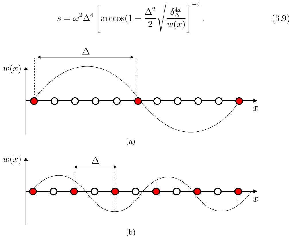
FIGURE 3.5 – Adaptation du pas \Delta dans le schéma aux différences finies de l'Équation (3.7) pour (a) une grande longueur d'onde et (b) une longueur d'onde plus faible. Le pas optimal est celui qui permet d'avoir trois points par longueur d'onde [65].
