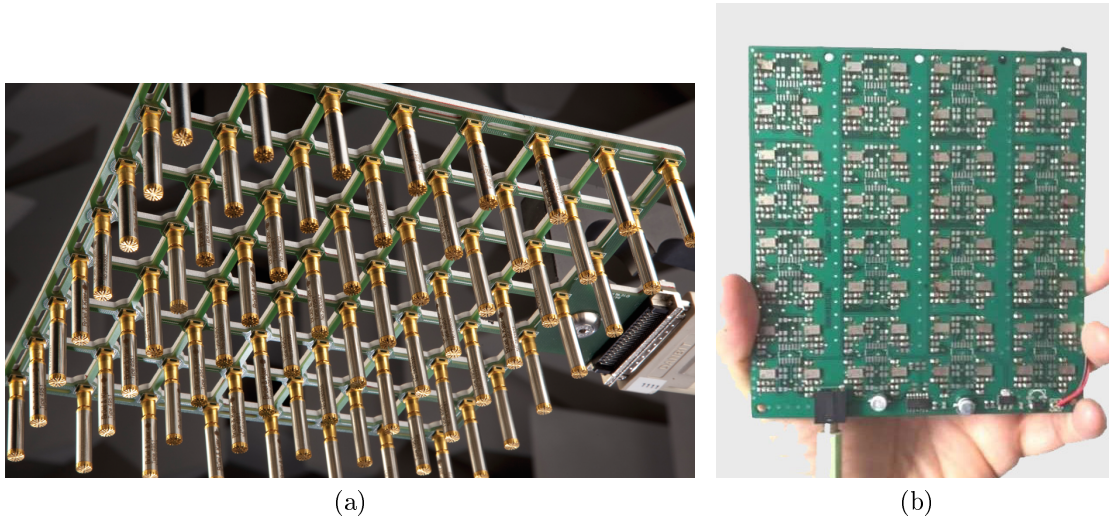
FIGURE 3.1 – (a) Réseau de microphones, image issue de Brüel and Kjær 1 , (b) Microphones sous formes de microsystèmes électromécaniques (MEMS), image issue de Dodotronic 2 . 1 bksv.com, 2 dodotronic.com
