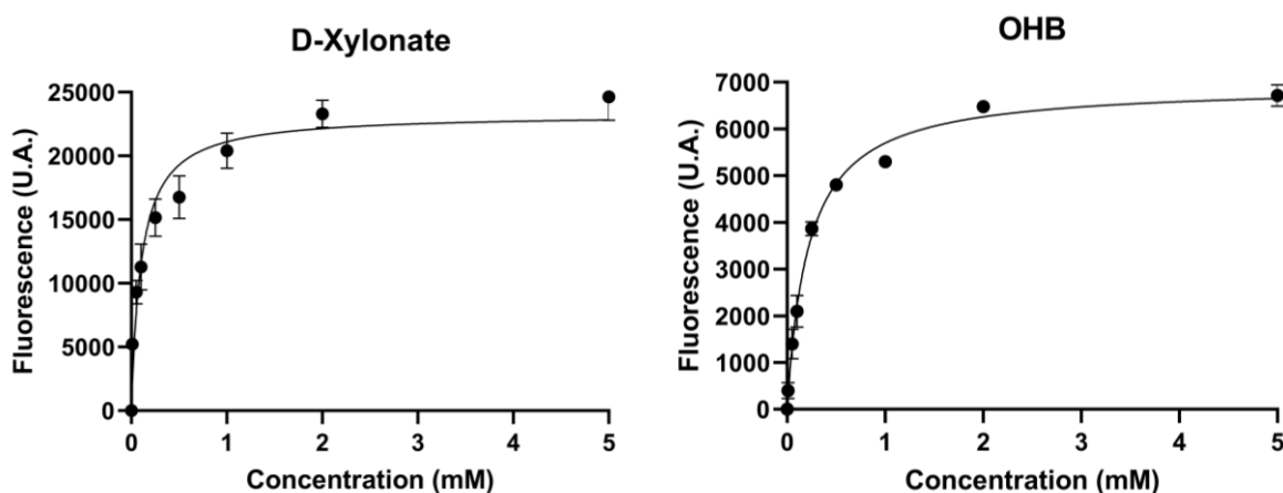
Figure 34 : Courbes d'affinité obtenues pour le D-xylonate et l'OHB. Les courbes en trait plein représentent la régression non linéaire (GraphPad, R^2 = 0.95 (D-xylonate) et 0.99 (OHB)).
