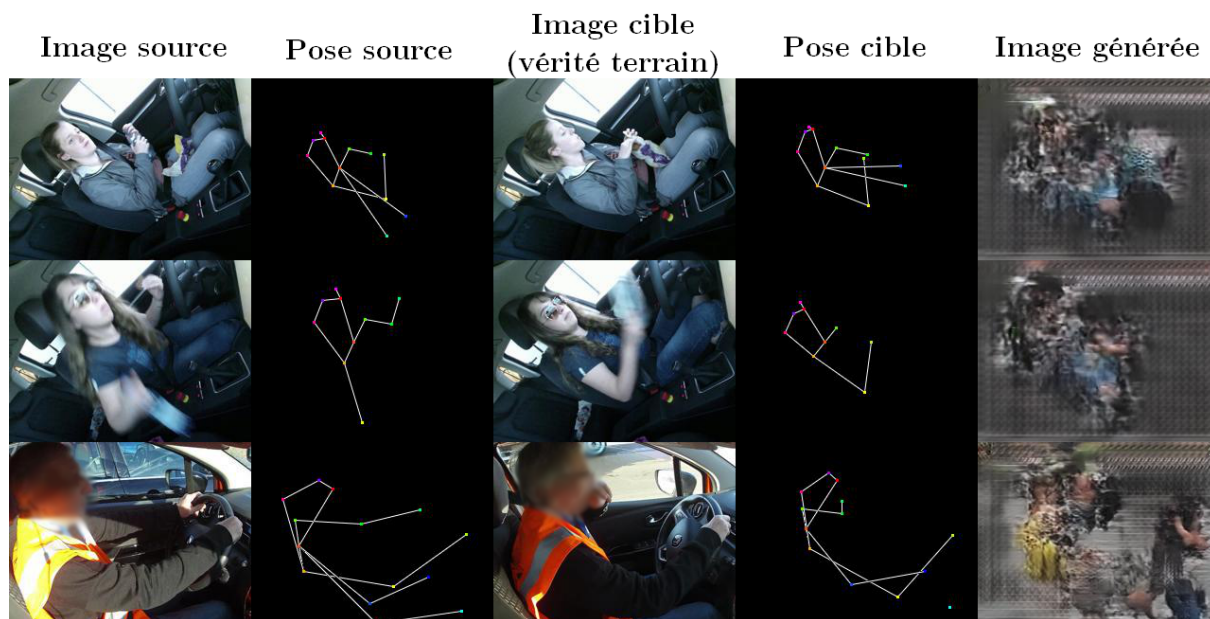
FIGURE 4.2 – Exemple d'inférence sur des images de conducteurs du réseau APS pré-entraîné sur Market-1501.
