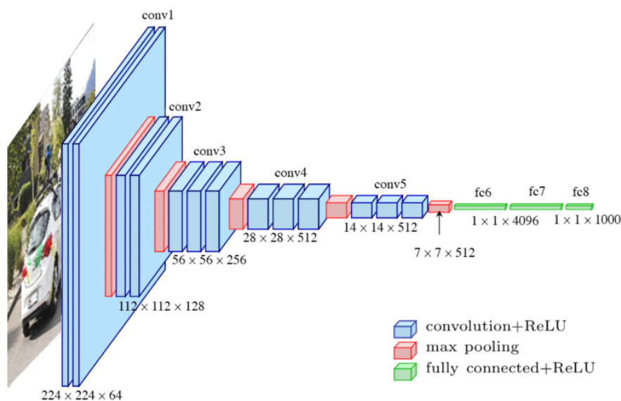
FIGURE 2.12 – Schéma de l'architecture VGG 16 (Ferguson et al., 2017).
