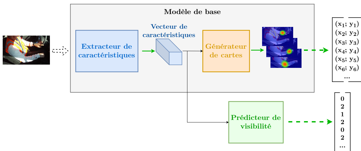
FIGURE 3.9 – Architecture du métamodèle multitâche proposé pour l'estimation de la pose et de la visibilité.
