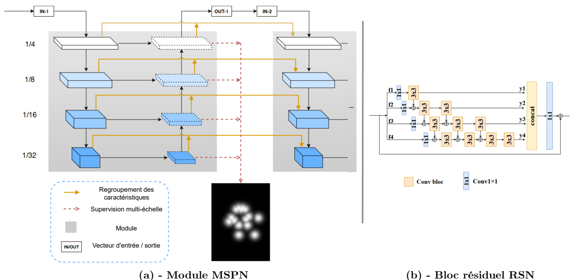
FIGURE 2.22 – Schémas d'un module de MSPN (a) (Li et al., 2019b) et d'un bloc résiduel de RSN (b) (Cai et al., 2020).
