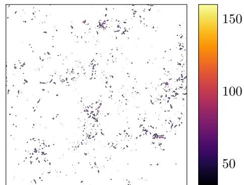
(d) \|\omega\|_2 > \langle \|\omega\|_2 \rangle_\Omega + 2\sigma(\|\omega\|_2)
