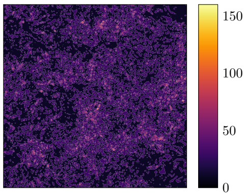
(c) \|\omega\|_2
