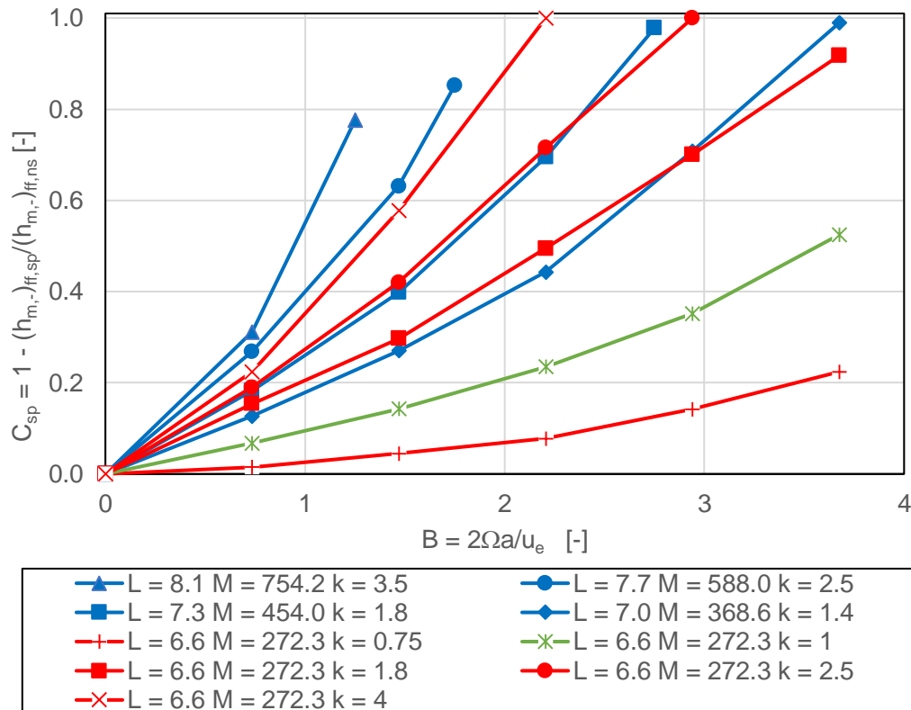
Figure 4.7. Influence du taux de pivotement/entraînement B sur l'épaisseur de film minimale pour différentes ellipticités k et conditions géométriques et de fonctionnement.
