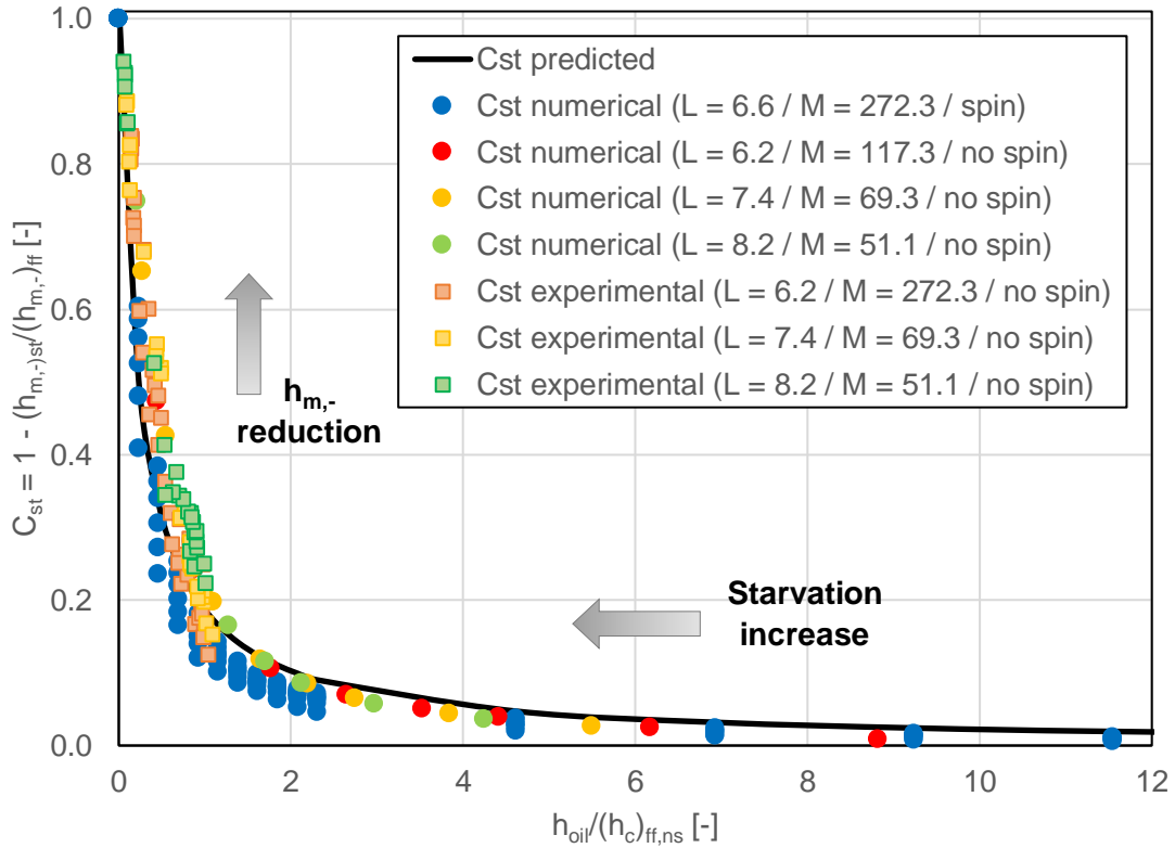
Figure 4.6. Variation de la réduction d'épaisseur de film critique C_{st} en fonction de la source d'alimentation en huile et pour différentes conditions de fonctionnement ( L et M ), avec et sans pivotement, obtenue à partir de simulations et d'expériences. Les flèches indiquent la direction croissante de la sous-alimentation et de la réduction de h_{m,-} .
