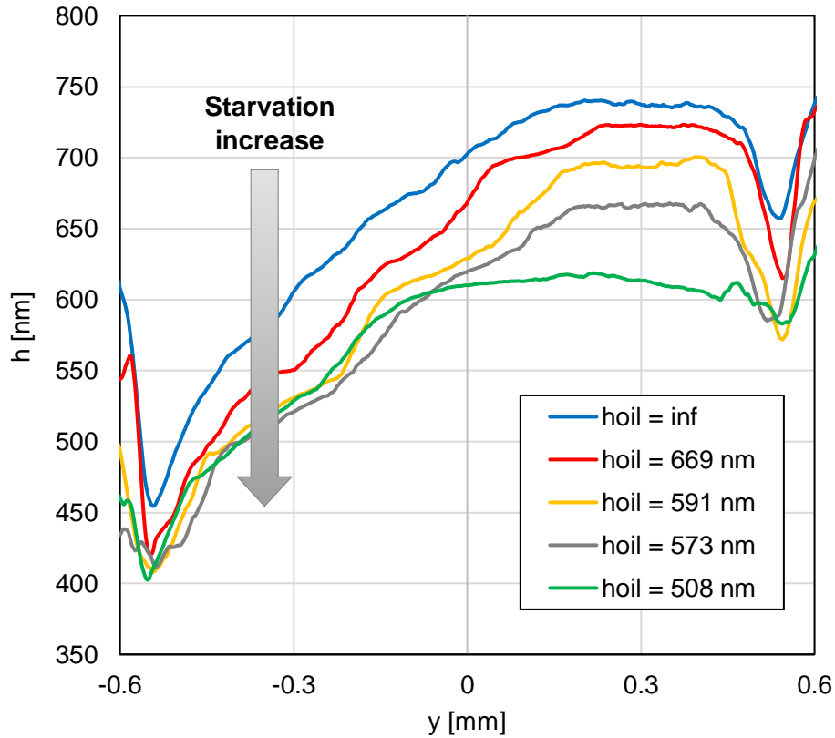
Figure 4.9. Profils d'épaisseur de film pour les interférogrammes a à e ( u_e = 0.5 m/s, w = 400 N, \Omega = 628 rad/s, \lambda = 0.8^\circ , T = 30^\circ\text{C} , R_x = R_y = 50 mm).
