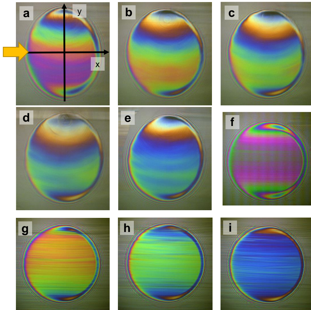
Figure 4.9. Interférogrammes obtenus avec Tribogyr. Les images a-e correspondent à des conditions de pivotement importantes ( \lambda = 0.8^\circ , avec h_{oil} = \text{inf}, 669, 591, 573, 508 \text{ nm} ) et les images f-i à des conditions de pivotement faibles ( \lambda = 9^\circ , avec h_{oil} = \text{inf}, 574, 464, 300 \text{ nm} ).
