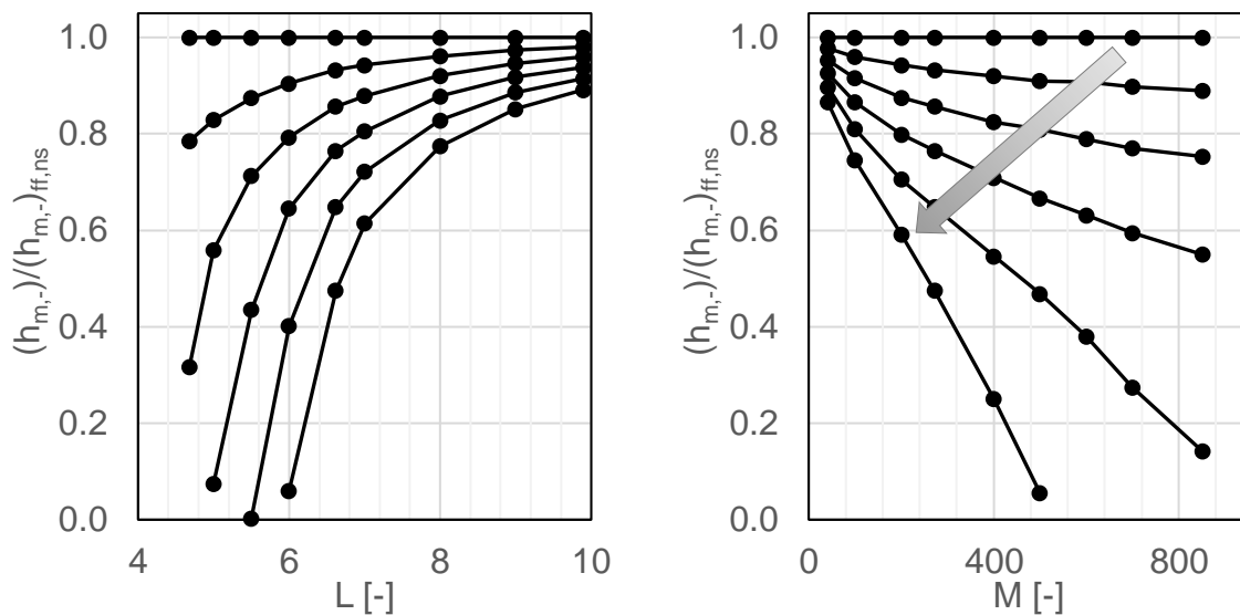
Figure 4.2. Variation de l'épaisseur de film minimale par rapport aux nombres sans dimensions L (gauche), avec M = 272 , et M (droit), avec L = 6.6 . Une flèche indique la direction de l'augmentation de la vitesse de pivotement.
