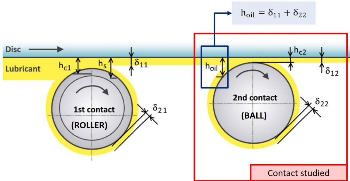
Figure 2.2. Représentation schématique du système rouleau-bille-disque (vue latérale).
