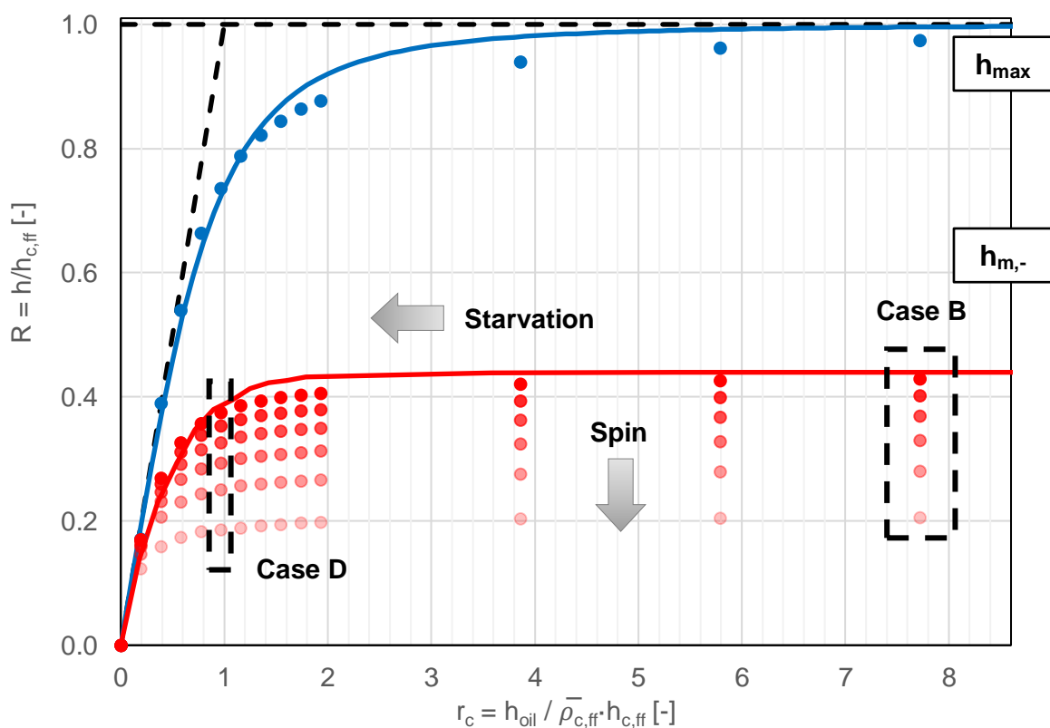
Figure 4.4. Variation des épaisseurs maximale ( R_{max} ) et minimale critique ( R_{m,-} ) sans dimension par rapport au réservoir d'huile sans dimension ( r_c ), pour des vitesses de pivotement différentes ( u_e = 2 m/s, w = 800 N, T = 30^\circ\text{C} , R_x = R_y = 80 mm).
