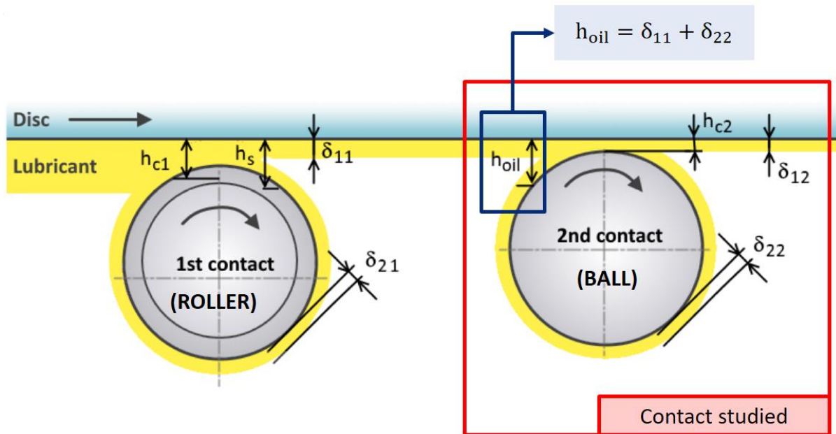
Figure 2.2. Représentation schématique du système roulement-bille-disque (vue latérale).
