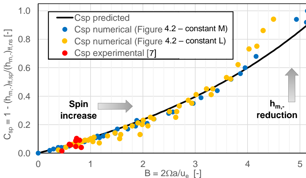
Figure 4.3. Effet du taux de pivotement/entraînement B sur l'épaisseur minimale critique du film pour différentes conditions de fonctionnement. Points expérimentaux calculés à partir des données extraites de [7].
