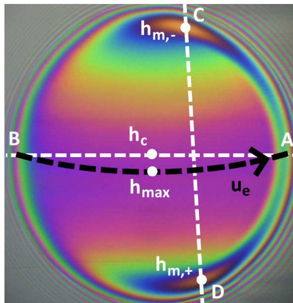
Figure 4.1. Épaisseurs de film représentatives dans un contact pivotant (interférogramme extrait de [7]). Le centre de rotation de l'éprouvette se trouve au-dessus de l'image.
