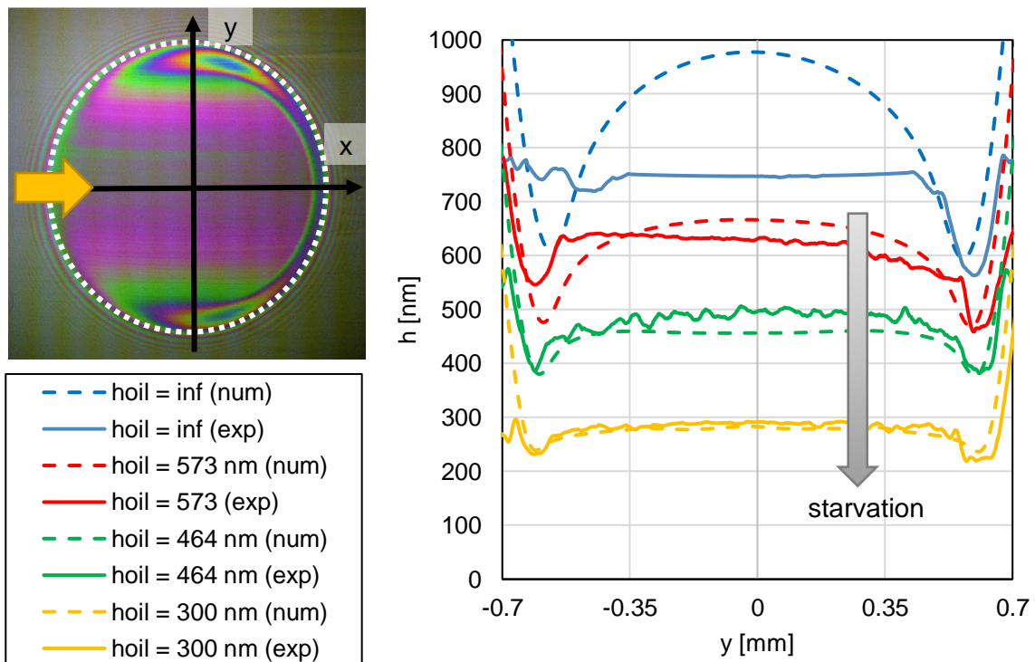
Figure 3.1. Épaisseurs du film le long de l'axe y pour u_e = 0.50 m / s et w = 400 N. La direction de la vitesse d'entraînement est représentée par une flèche jaune. L'interférogramme (à gauche) correspond au cas suralimenté. La zone de contact hertzienne est marquée par un cercle en pointillé.
