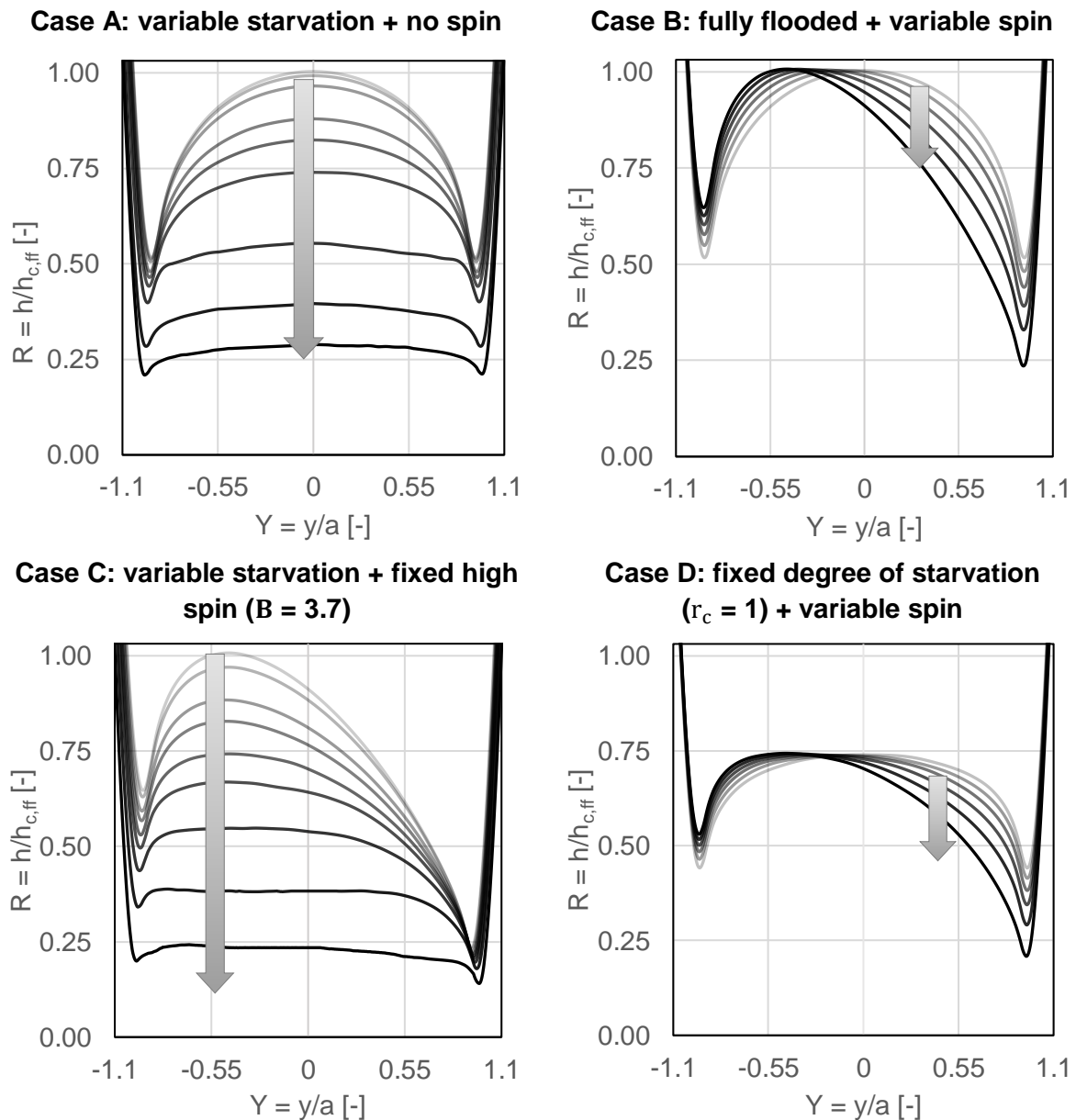
Figure 4.5. Profils d'épaisseur de film transversaux pour différents cas d'étude extraits de la Figure 4.4. Les flèches indiquent la direction croissante de pivotement (cas B et D) ou de degré de sous-alimentation (cas A et C).
