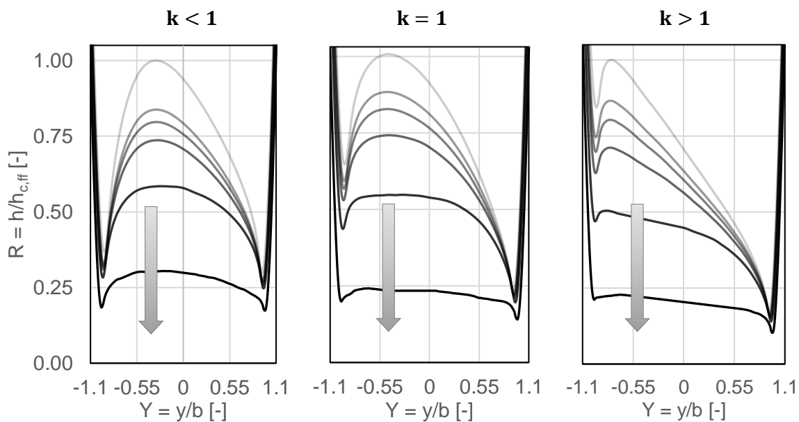
Figure 4.8. Profils d'épaisseur de film transversaux pour différents rapports d'ellipticité ( k = 0.75, 1, 1.8 ) et des conditions de pivotement et de lubrification identiques ( u_e = 2 m/s, w = 800 N, T = 30^\circ\text{C} , R_x = 80 mm, \Omega = 4000 rad/s). Une flèche illustre la direction des degrés de sous-alimentation croissants.
