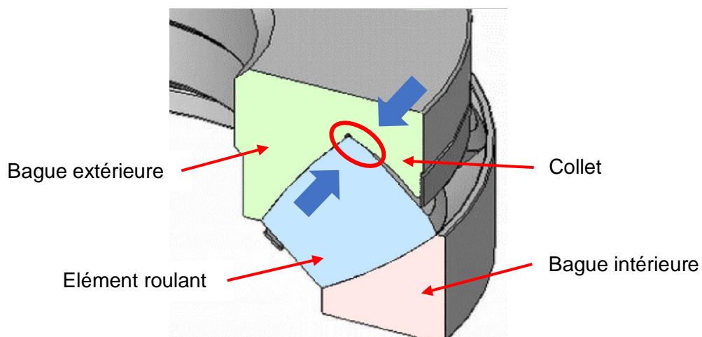
Figure 1.1. Emplacement du contact rouleau/collet (marqué par une ellipse rouge) dans un roulement conique. Les flèches bleues indiquent la charge exercée par les deux éléments en contact.
