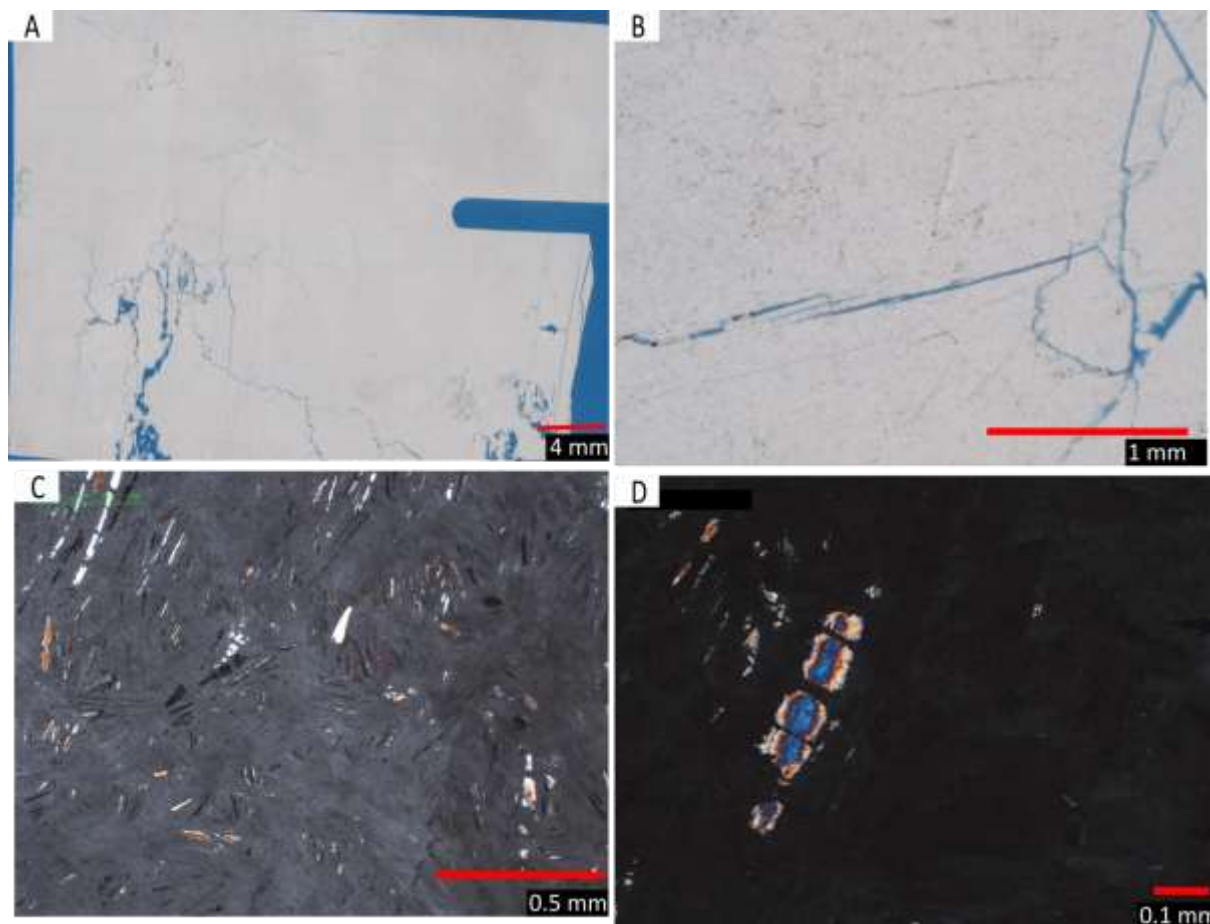
Figure 124 Observation au microscope optique de lame mince pétrographique réalisée sur un échantillon de gypse albaströide. A : vue générale du gypse albaströide (x 20). B : Porosité fissurale du gypse albaströide (x20), C : zone contenant des minéraux polarisant dans les teintes du 3 ème ordre pris dans le gypse albaströide (x50, LPA). D : minéral inclus dans la masse de gypse (x100 LPA)
