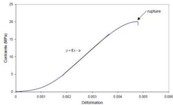
Figure 104 Exemple de courbe contrainte déformation. (Tomachot, 2002)
