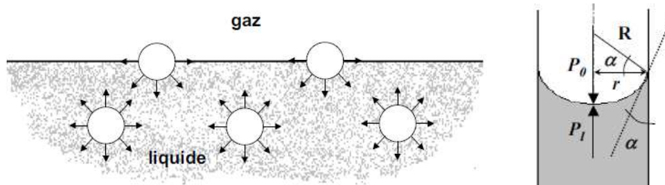
Figure 101 Représentation schématique de la tension interfaciale à l'interface liquide-gaz. (Rousset-Tournier, 2001)
