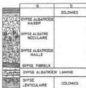
Figure 80 Log stratigraphique des gypses du Lutétien supérieur (Toulemont, 1986)
