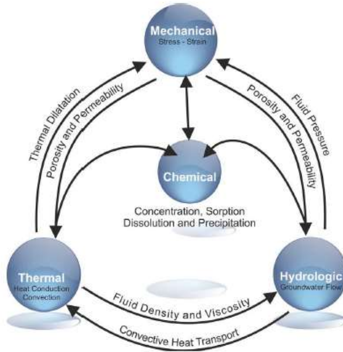
Figure 66 Relations dans les couplages THMC. (Rühaak et al., 2015)
