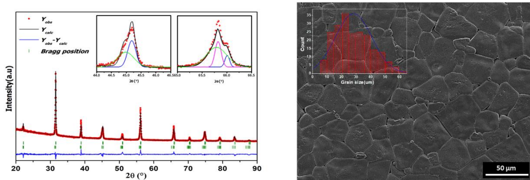
Figure 1 : (a) Diagrammes de diffraction des rayons X de la céramique BCTSn ; (b) Micrographie MEB de la céramique BCTSn, l'encart de la figure montre la distribution granulométrique.
