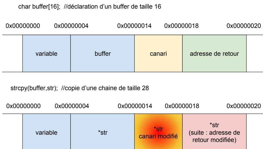
FIGURE 2.7 – Mécanisme de protection de type canari
