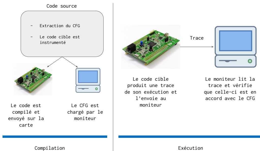
FIGURE 3.3 – Fonctionnement général
