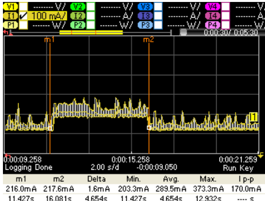
(a) Envoi de 2 paquets de données de 400 Octets chacun. Energie consommée équivalente à 12 Joules.
