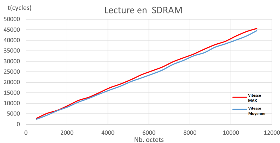
FIGURE 5.10 – Quantification de la vitesse de lecture en SDRAM en fonction de la taille des données à lire.
