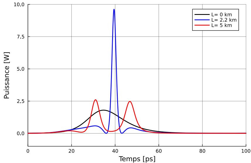
FIGURE 4.29 – Comparaison du signal laser à différentes distances dans la fibre optique. Puissance moyenne en entrée : 400 mW.
