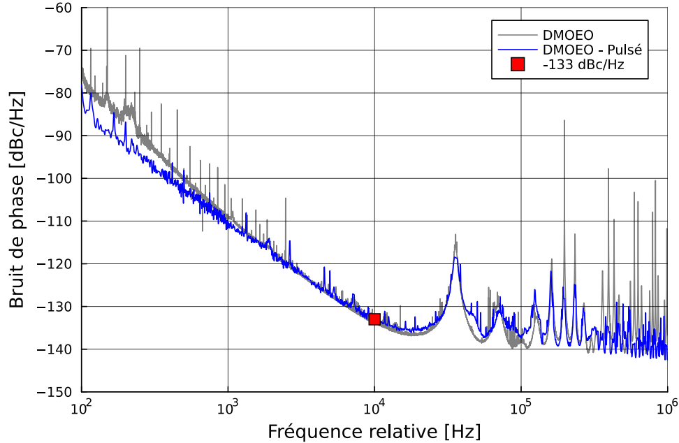
FIGURE 4.21 – Bruit de phase du DMOEO à compression d'impulsion.
