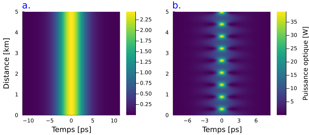
FIGURE 4.9 – Simulation de solitons dans une fibre standard de 5 km. a. Soliton fondamental ( N = 1 , \Delta\tau = 5 ps, P = 2.4 W), b. Soliton d’ordre 2 ( N = 2 , \Delta\tau = 5 ps, P = 9.7 W).
