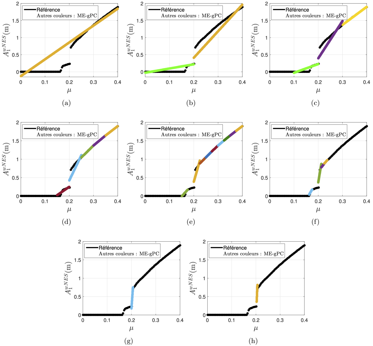
FIGURE 1.28. Huit itérations jusqu'à l'arrêt de l'algorithme de la Fig. F.4 pour la détection de la limite d'atténuation.
