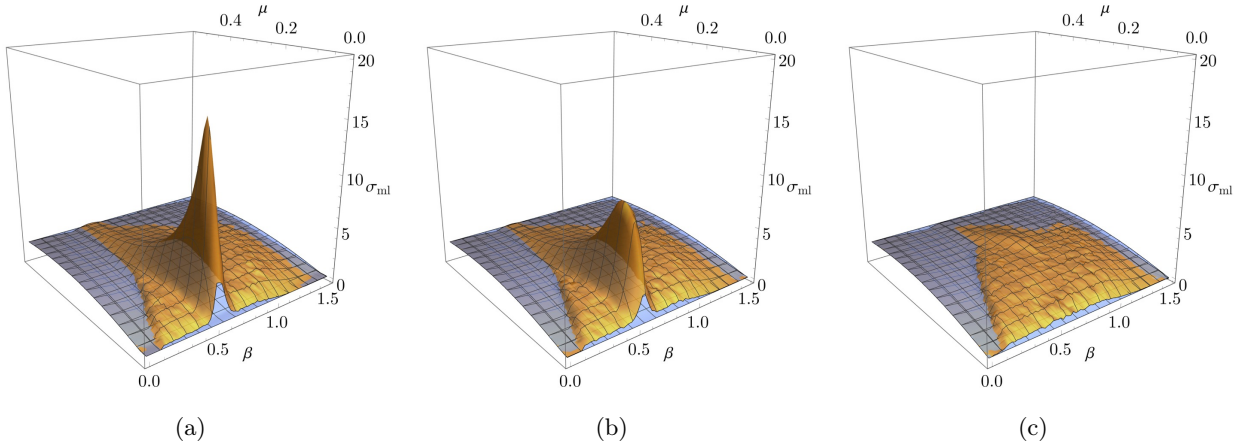
FIGURE 1.12. Limite d'atténuation \sigma_{\text{ml}} , en fonction de \beta et \mu , d'un NES (surface bleue) et d'un BNES (surface orange). Les conditions initiales sont (x_0, y_0) = p_0^{\text{st}} + (\text{per}, \text{per}) pour le NES et (x_0, y_0) = p_1^{\text{st}} + (\text{per}, \text{per}) pour le BNES, respectivement. Le paramètre de perturbation est \text{per} = 0.001, 0.01 et 0.1 dans (a) à (c), respectivement.
