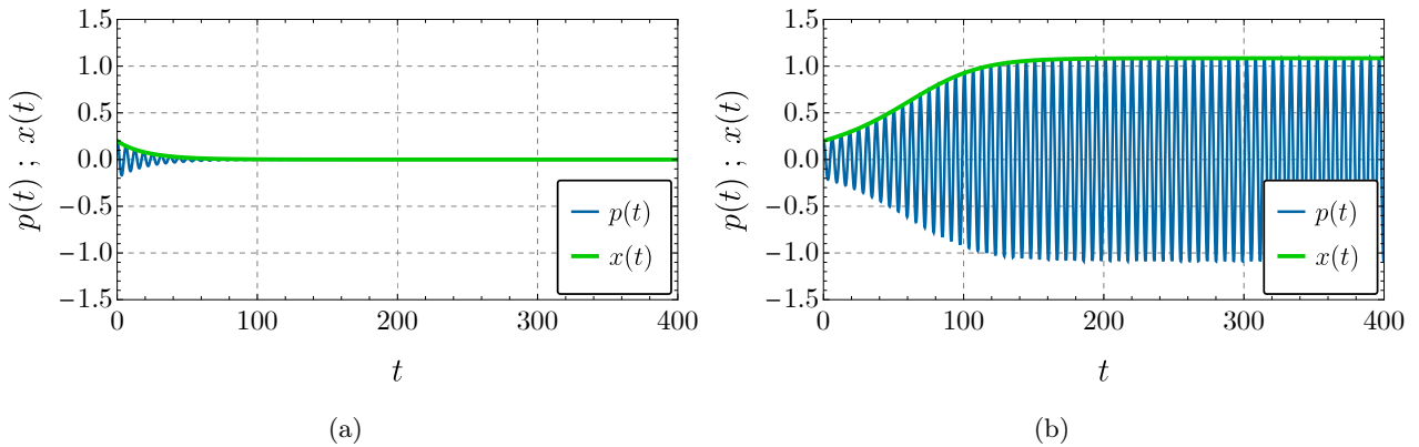
FIGURE 2.6. Exemples d'intégration numérique des Éqs. (2.48) et (2.50) : series temporelle de x(t) (vert) et p(t) (en bleu). Mêmes paramètres qu'en Fig. 2.5 avec (a) \gamma = 0.2 < \hat{\gamma}^{\text{st}} (c.-à-d. la solution triviale est stable) et (b) \gamma = 0.6 > \hat{\gamma}^{\text{st}} (c.-à-d. la solution triviale est instable et la solution périodique est stable).
