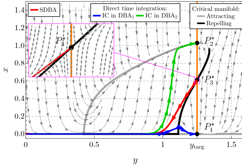
FIGURE 2.18. Figure similaire à la Fig. 2.17(a). En rouge, une orbite obtenue par l'intégration numérique du système a temps inversé (2.87) avec g(y) = y_{\text{targ}} - y et une condition initiale (CI) choisie comme une petite perturbation du point fixe non trivial P_3^* . En bleu et vert, deux orbites obtenues par l'intégration de l'Éq. (2.89) : avec une CI d'abord dans le \text{DBA}_1 (en bleu) et dans le \text{DBA}_2 (en vert). Les lignes de courant de l'Éq. (2.89) (lignes fléchées grises) sont également représentées.
