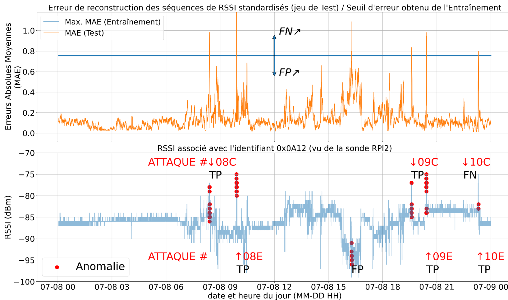
Figure 6-9. Détection d'usurpation d'identité par auto-encodeur à cellules LSTM exploitant des séquences de RSSI (sonde RPI2, identifiant 0x0A12), journée avec 6 attaques du 8 juillet 2022
