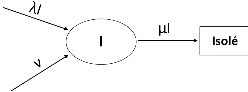
FIGURE 3.1 – Modèle à un seul compartiment : Infecté.
