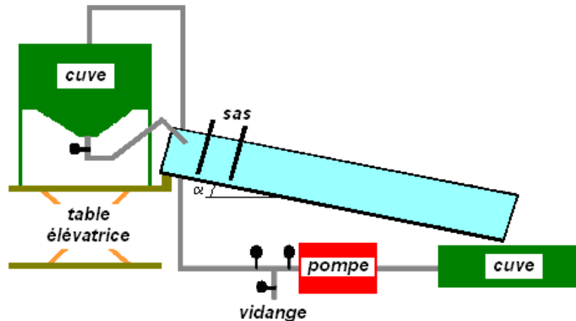
Figure 5.11 Canal expérimental
