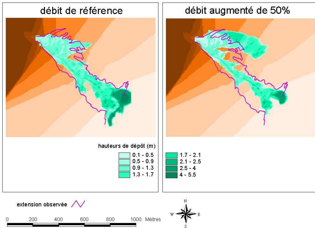
Figure 3.10 Sensibilité du modèle aux variations du débit entrant (Varunasch), hypothèses retenues pour la simulation : volume = 215 000 m 3 , \tau_c/\rho = 1,8 \text{ m}^2\text{s}^{-2} , K/\tau_c = 0,3 \text{ s}^{1/3} , grille de calcul constituée de cellules carrées de 5 m de côté.
