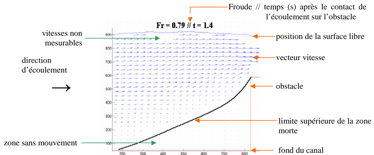
Figure 5.14 Données générales sur l'écoulement en amont de l'obstacle, les axes sont en pixels (1 pixel = 0,007 cm), l'origine des temps correspond au premier contact de l'écoulement sur l'obstacle.
