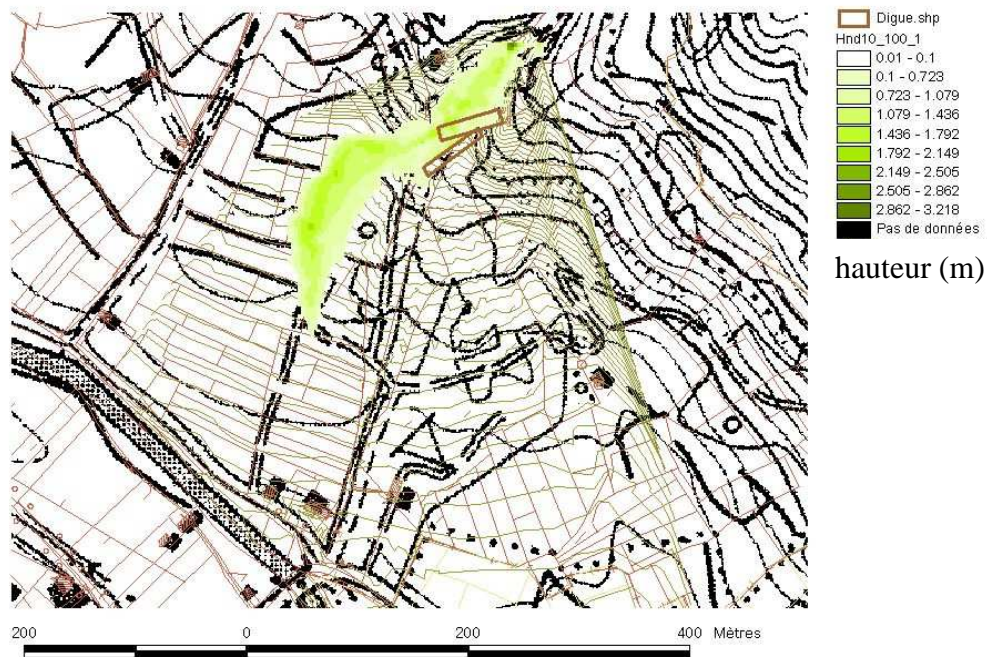
Figure 4.19 Hauteurs maximales simulées pour un volume de 10\,000\text{ m}^3 , un débit de pointe de 100\text{ m}^3/\text{s} et un rapport \tau_c/\rho = 1,0\text{ m}^2/\text{s}^2 dans l'hypothèse de l'implantation d'une digue présentant un angle d'incidence d'environ 15^\circ par rapport au chenal amont du torrent
