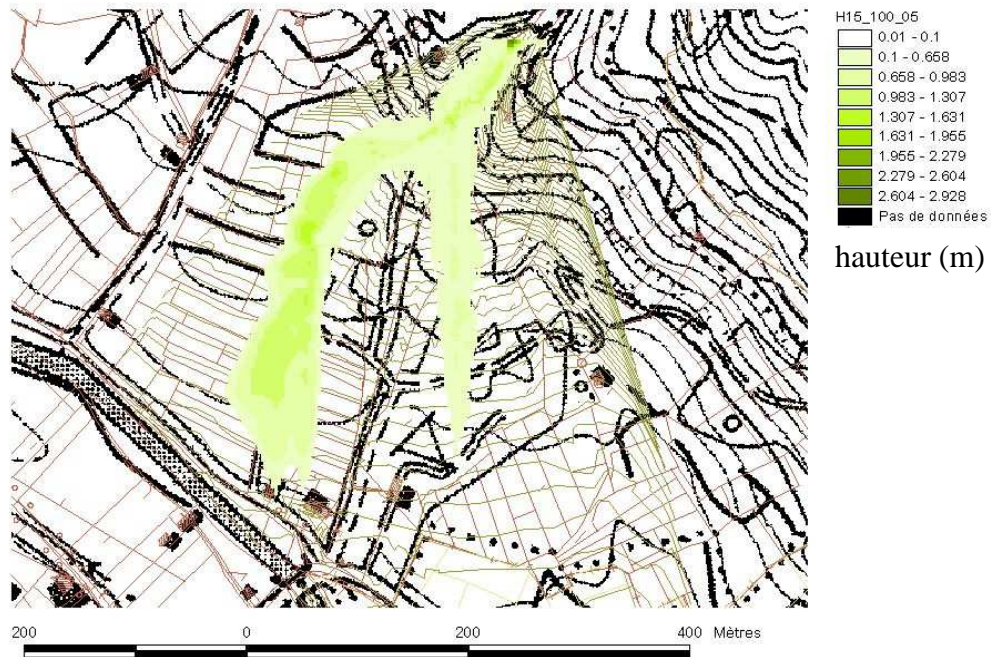
Figure 4.13 Hauteurs maximales simulées pour un volume de 15 000 m 3 , un débit de pointe de 100 m 3 /s et un rapport \tau_c/\rho = 0,5 \text{ m}^2/\text{s}^2
